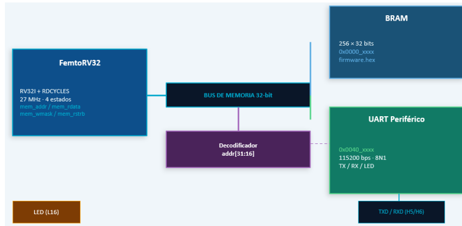
Figura 1: Diagrama de bloques del SoC Femto. La CPU genera direcciones hacia el multiplexor de decodificación, que activa bram_cs o uart_cs según el rango. Los datos de lectura retornan por mem_rdata y los de escritura viajan por mem_wdata .
