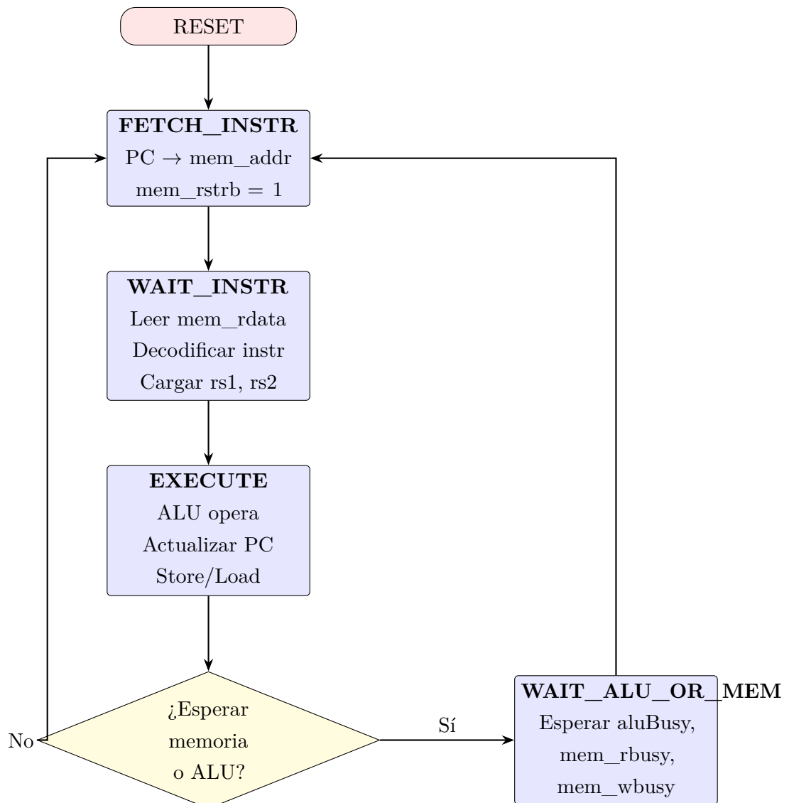
Figura 2: Máquina de estados del procesador FemtoRV32.
