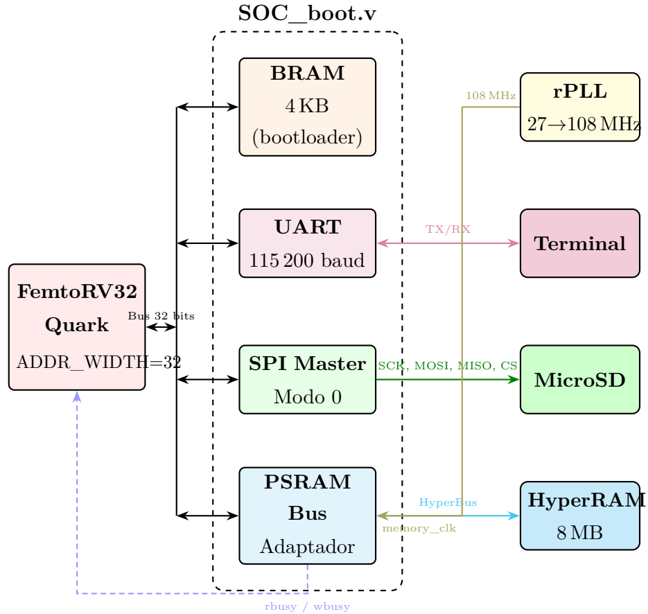
Figura 4: Arquitectura expandida del SoC FemtoUN Boot. Se añaden el controlador SPI para lectura de MicroSD, el adaptador de bus PSRAM para acceso a HyperRAM de 8 MB, y un PLL que genera los 108 MHz requeridos por la PSRAM.
