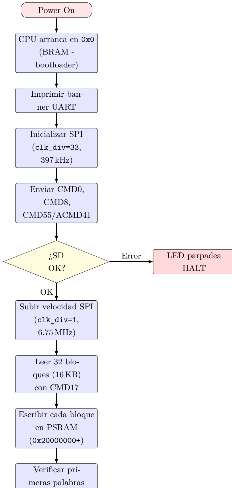
Figura 5: Flujo de arranque del bootloader FemtoUN Boot.
