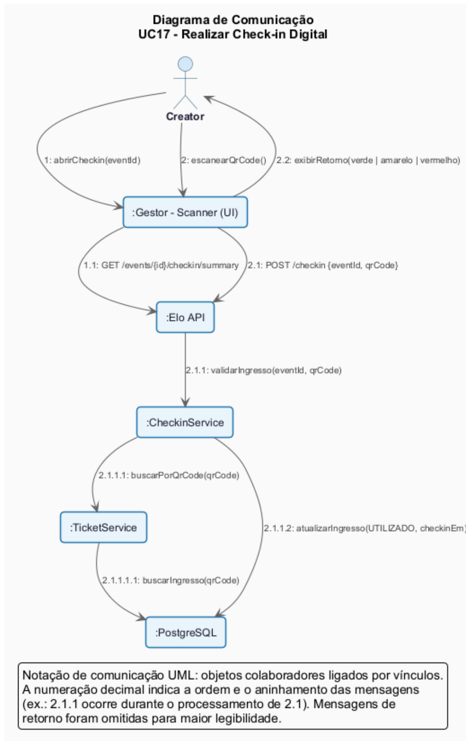
Figura 14: Diagrama de Comunicação: UC17 Check-in.
