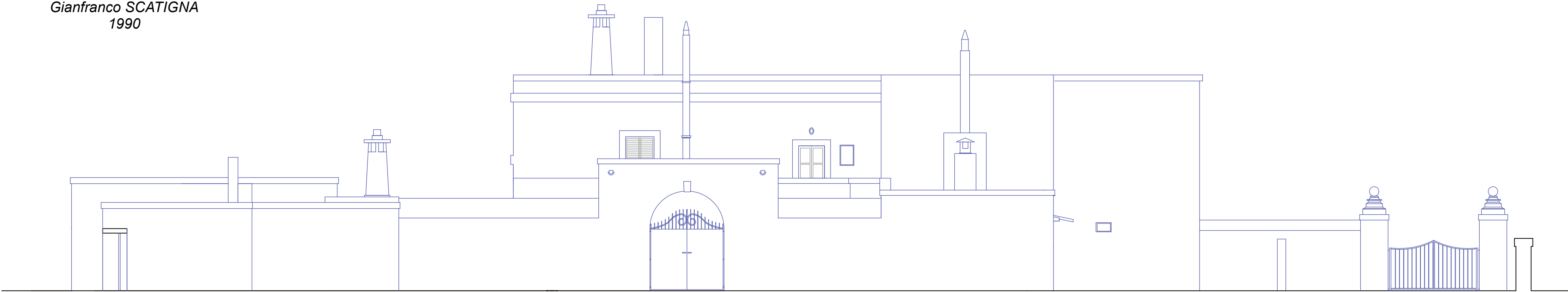
PROSPETTO ARCO D'INGRESSO CORTE - Scala 1:100
