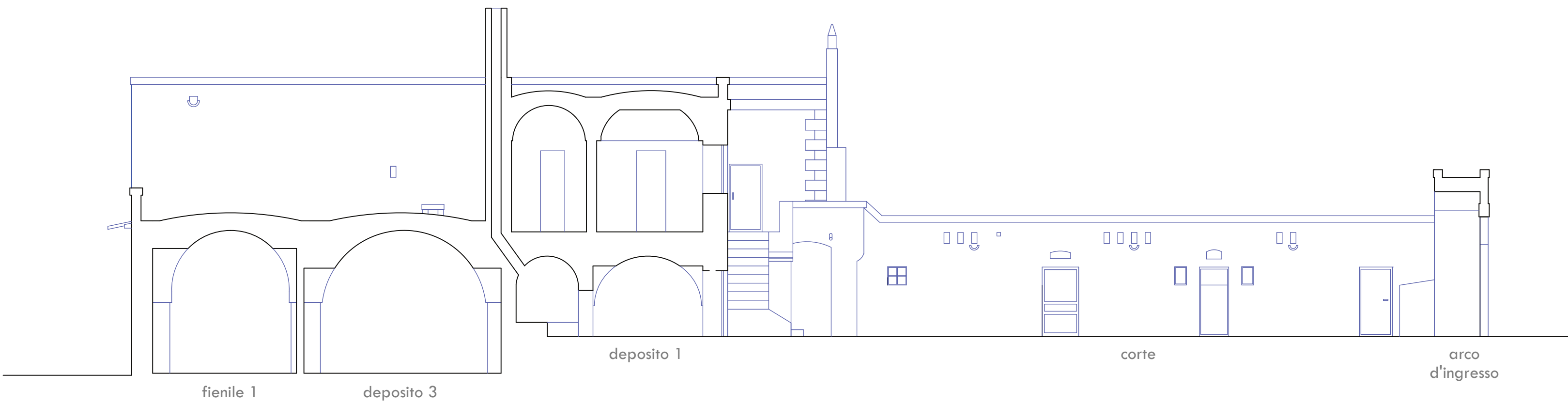
SEZIONE 3-3 VERSO STALLA BOVINI - Scala 1:100
