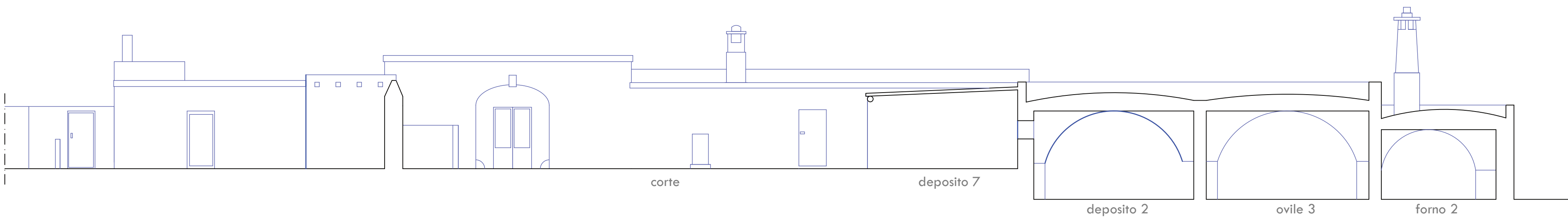
SEZIONE 4-4 VERSO STALLE CAVALLI E OVINI - Scala 1:100
