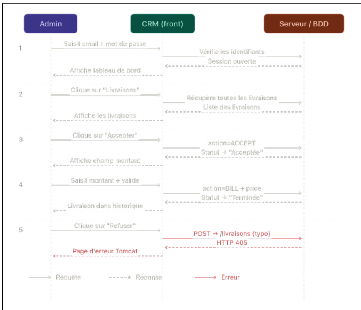
Diagramme de séquence Admin
