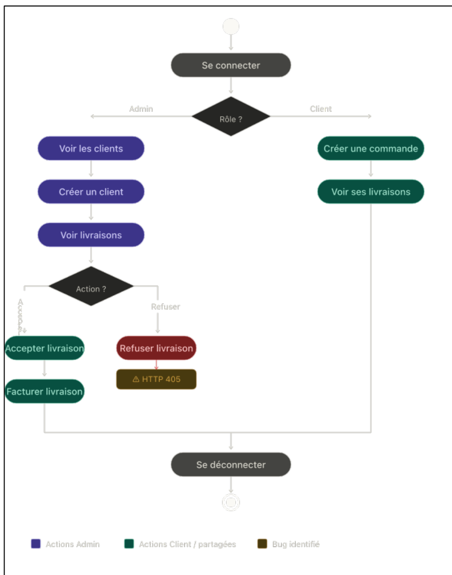
Diagramme d'activité
