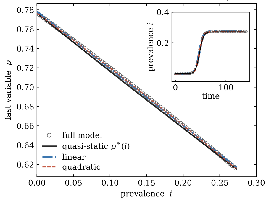
Pairwise SIS
