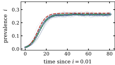
Pairwise SIS
