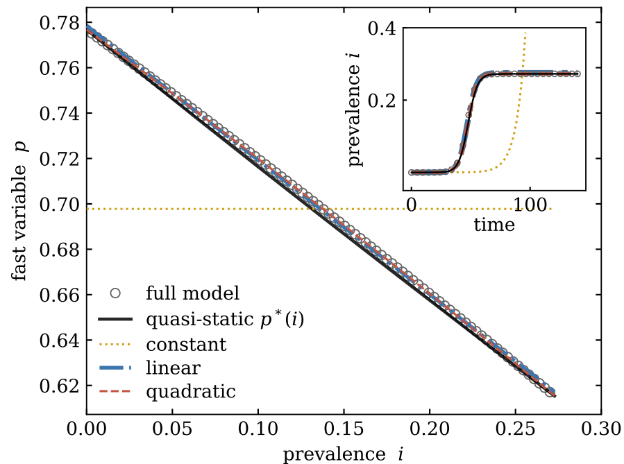
Pairwise SIS
