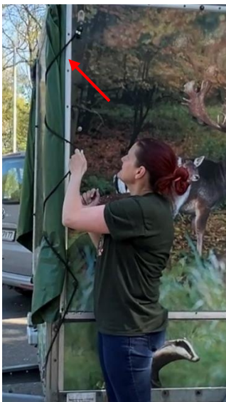
Gummis an allen 4 Ecken lösen
