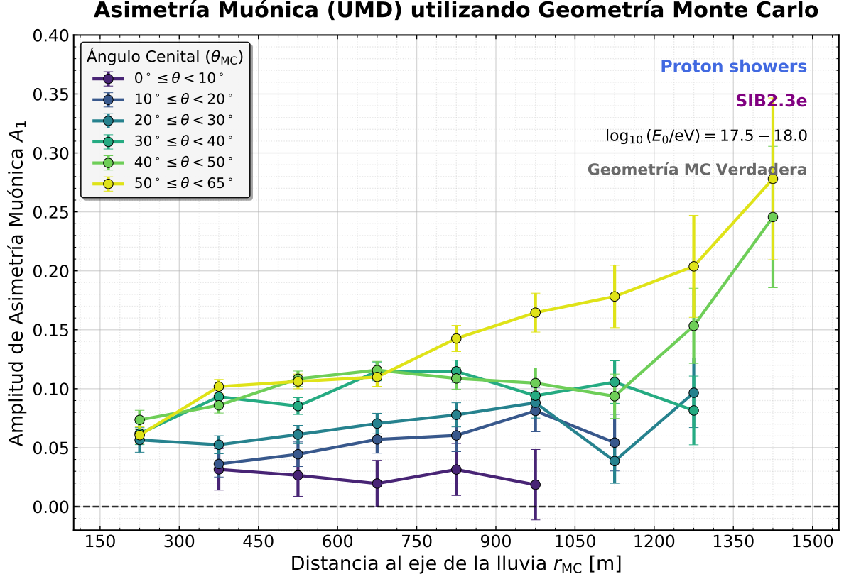
Figura 6.1: Evolución radial de A_1 en el UMD para distintas inclinaciones, con geometría Monte Carlo. Se conservan las condiciones de selección de la muestra original. Los intervalos mostrados no constituyen una medición de una población UMD previa a toda selección instrumental.
