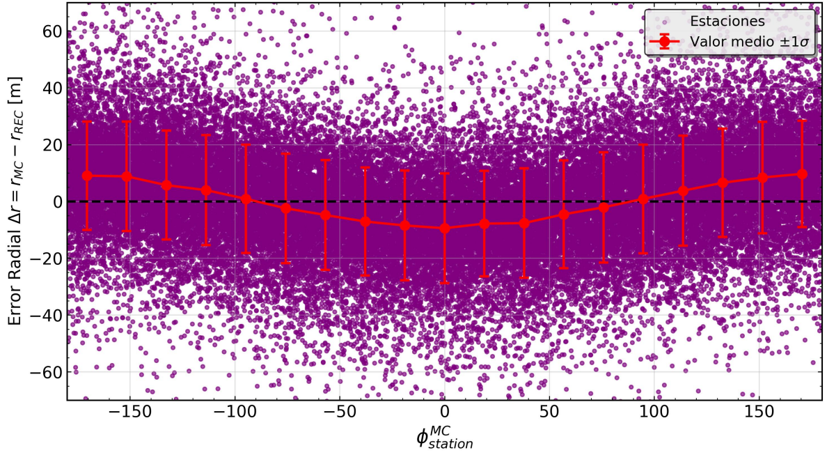
Figura 5.7: Distorsión de la coordenada radial de las estaciones del Infill en función del ángulo azimuthal. La modulación es compatible con un componente sistemático del error geométrico a lo largo del eje temprano–tardío; no identifica por sí sola su origen.
