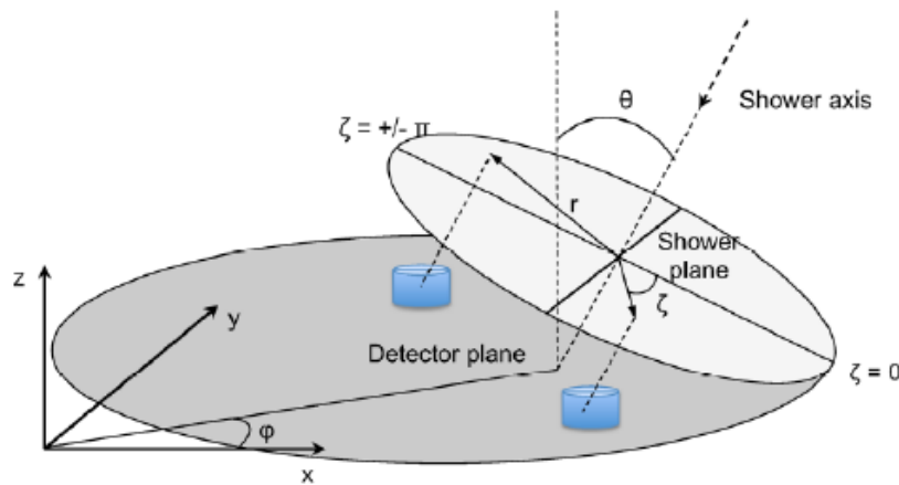
Figura 3.1: Proyección de las posiciones del suelo al plano perpendicular al eje de la lluvia. El azimut indicado como \zeta en el esquema corresponde a \phi en este trabajo.
