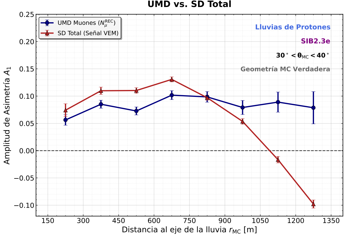
Figura 6.3: UMD frente a señal total SD para 30^\circ \leq \theta < 40^\circ , utilizando geometría Monte Carlo. La inversión de la señal SD se observa dentro de la selección original de estaciones. Los dos detectores no miden la misma población ni la misma magnitud física.
