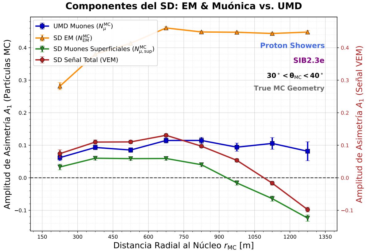
Figura 6.4: Desglose de la asimetría azimuthal para las componentes inyectadas a nivel del suelo frente a la respuesta del detector subterráneo ( 30^\circ \leq \theta < 40^\circ ). La asimetría electromagnética del SD (naranja) exhibe un comportamiento marcadamente positivo acoplado a la evolución longitudinal. En contraste, los muones superficiales del SD (verde) presentan una asimetría negativa a grandes distancias, producto del efecto de dispersión geométrica por proyección del disco [5].
