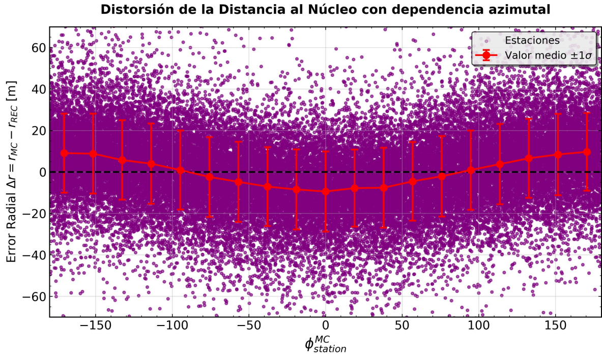
Figura 5.7: Distorsión de la coordenada radial de las estaciones del Infill en función del ángulo azimuthal. La modulación armónica demuestra que el núcleo reconstruido no sufre un espaciamiento aleatorio, sino un corrimiento sistemático a lo largo del eje temprano-tardío.
