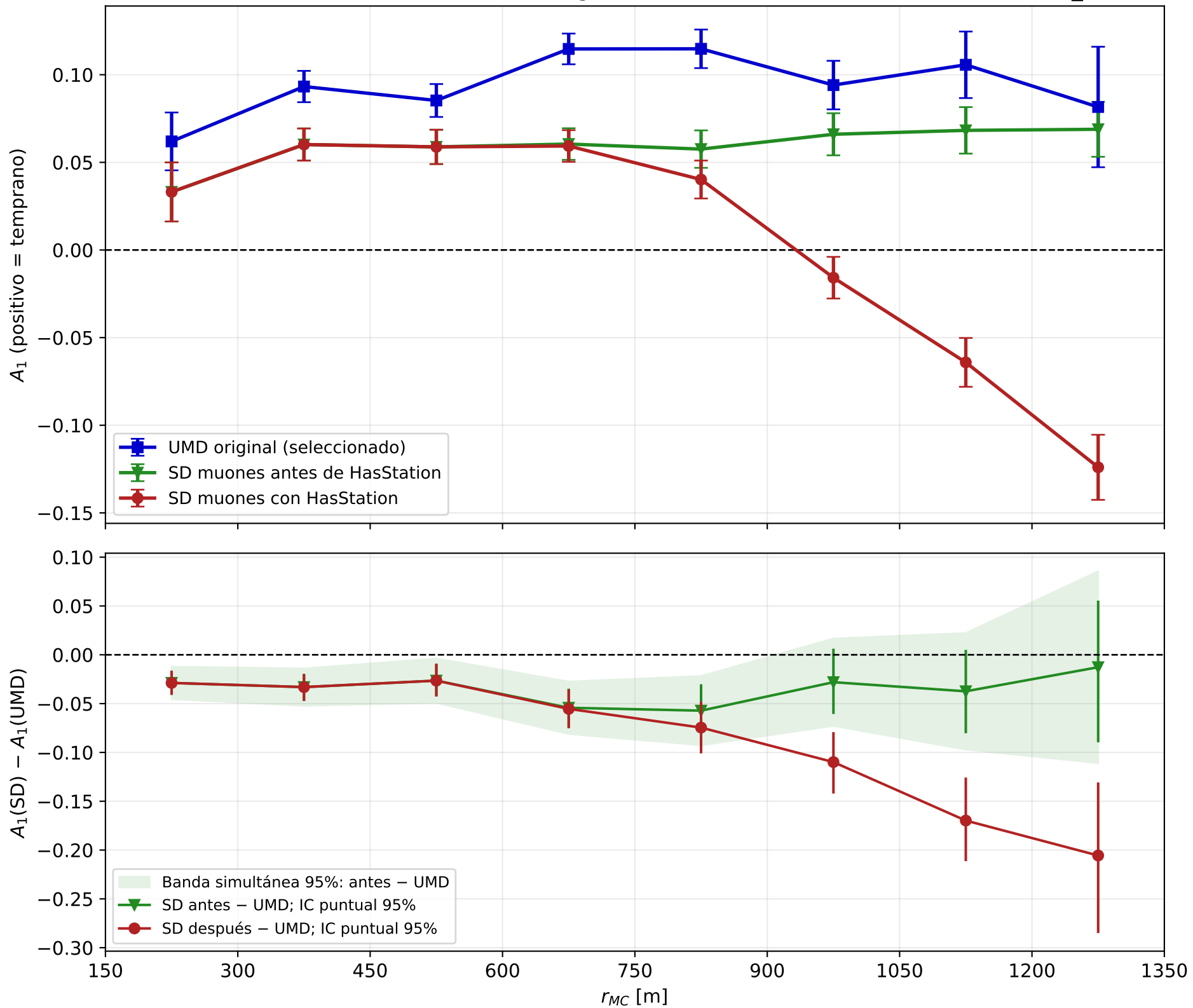
¿El SD antes del corte reproduce la asimetría UMD? Protones SIBYLL 2.3e; 30 \leq \theta_{MC} < 40^\circ ; geometría MC verdadera — fuente: insumos_astra
