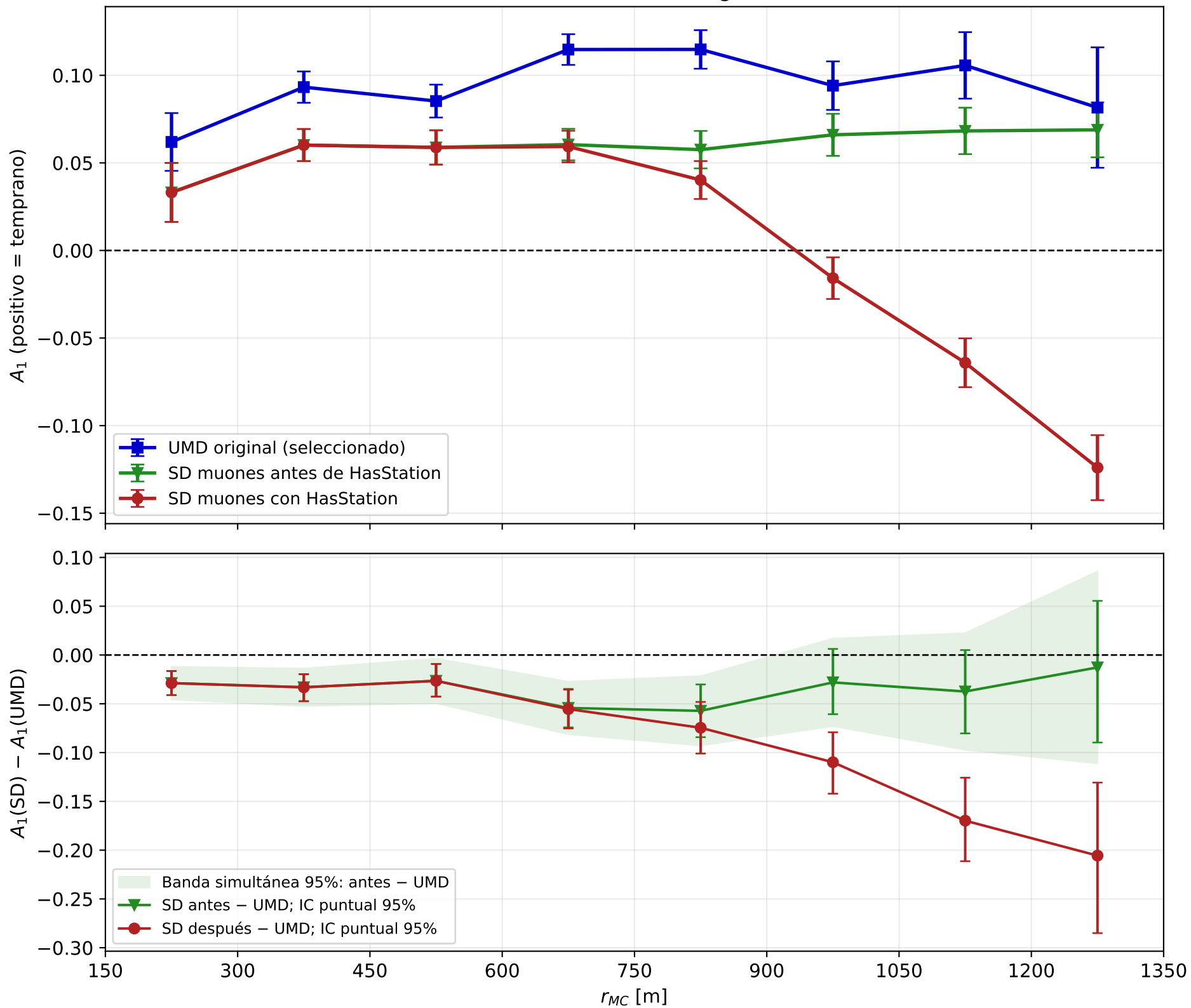
¿El SD antes del corte reproduce la asimetría UMD? Protones SIBYLL 2.3e; 30 \leq \theta_{MC} < 40^\circ ; geometría MC verdadera
