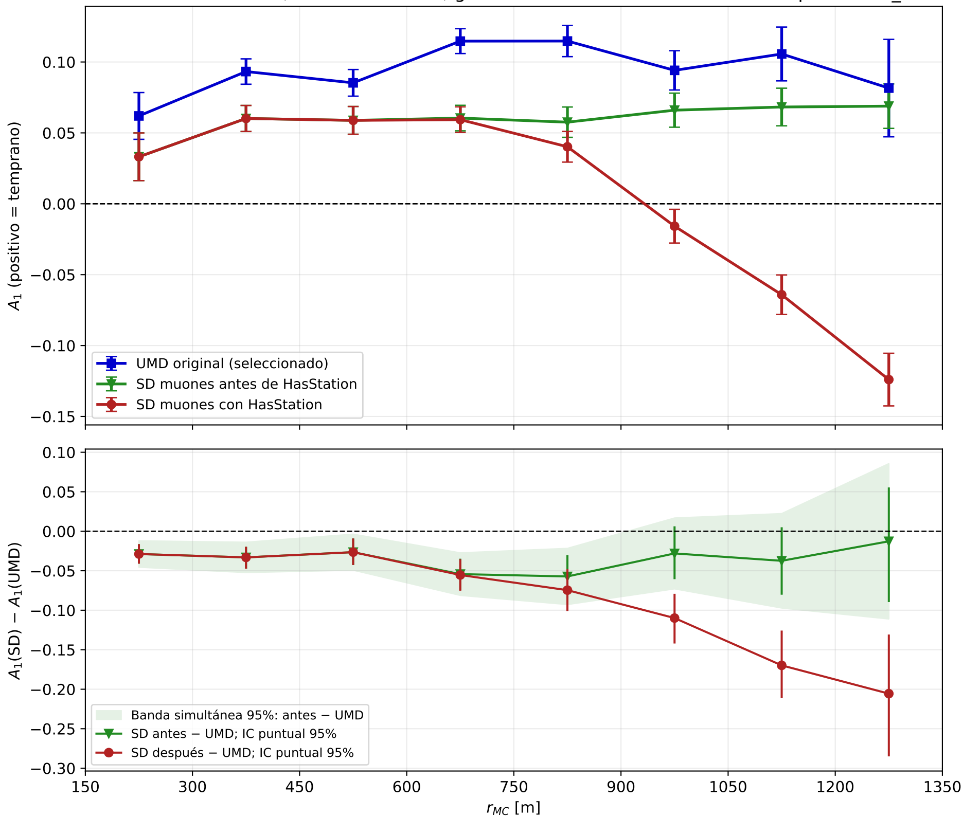
¿El SD antes del corte reproduce la asimetría UMD? Protones SIBYLL 2.3e; 30 \leq \theta_{MC} < 40^\circ ; geometría MC verdadera — fuente: reprocesado_v13
