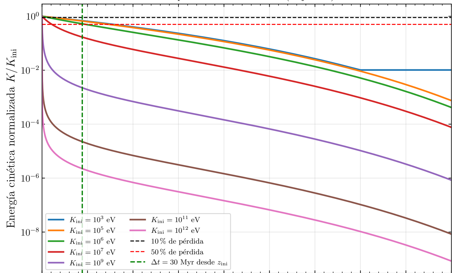
Compton inverso sobre el CMB ( z dinámico)
