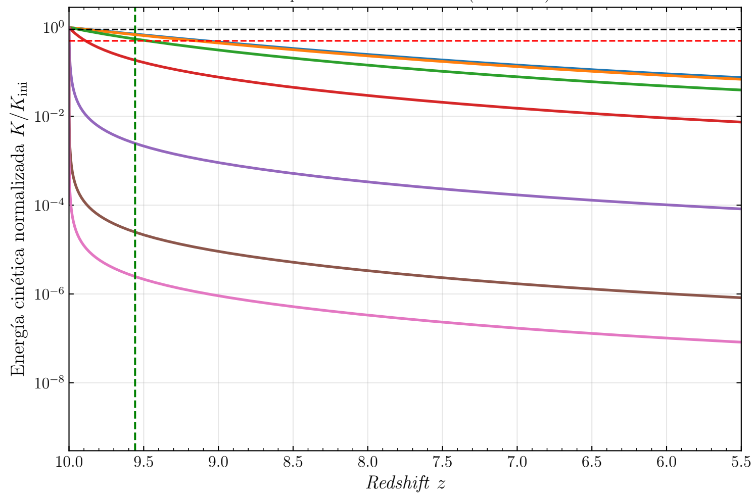
Compton inverso sobre el CMB ( z dinámico)
