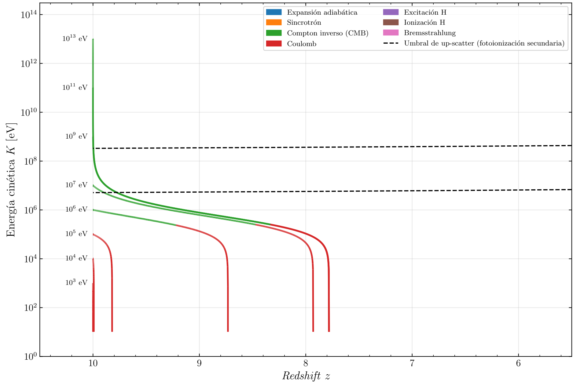
Todos los mecanismos de pérdida activos, x_e = 0.5
