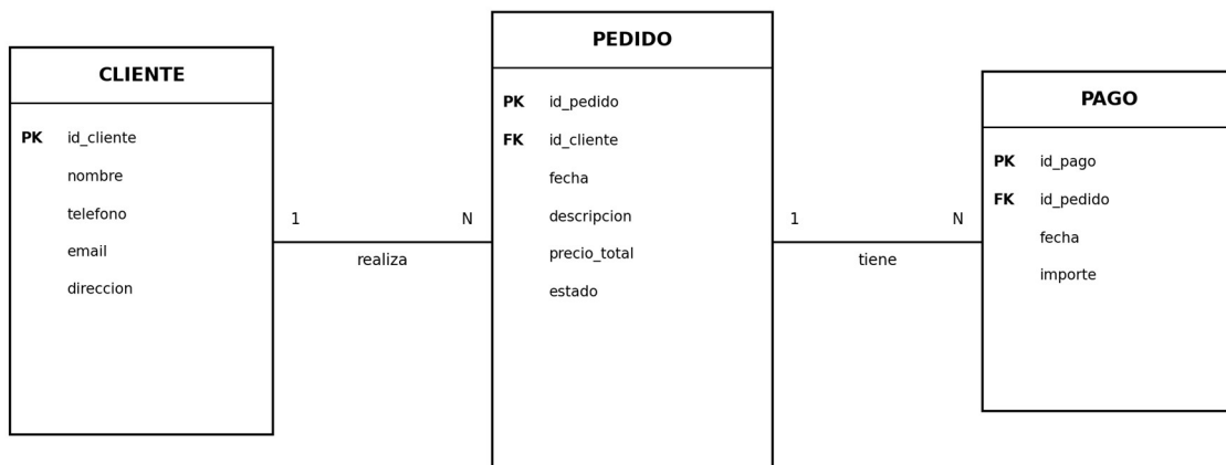
Figura 3 - Modelo Entidad-Relación
