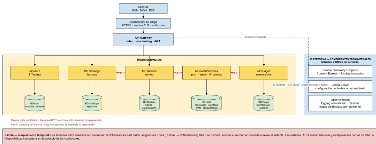
Figura 2 – Paso A: microservicios tradicionales con comunicación REST síncrona
