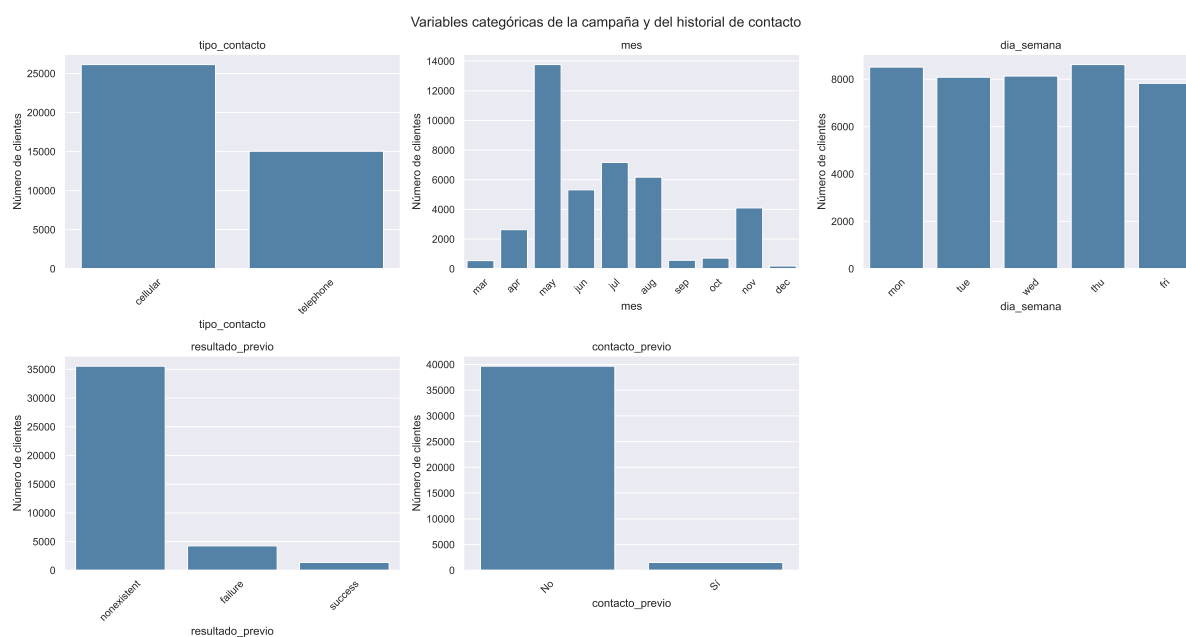
Figura 7: Gráficos de barras de las variables categóricas de la campaña y del historial de contacto.
