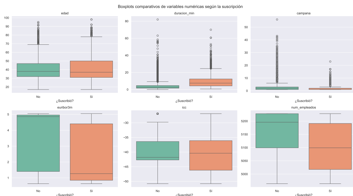
Figura 9: Boxplots comparativos de variables numéricas según la suscripción.
