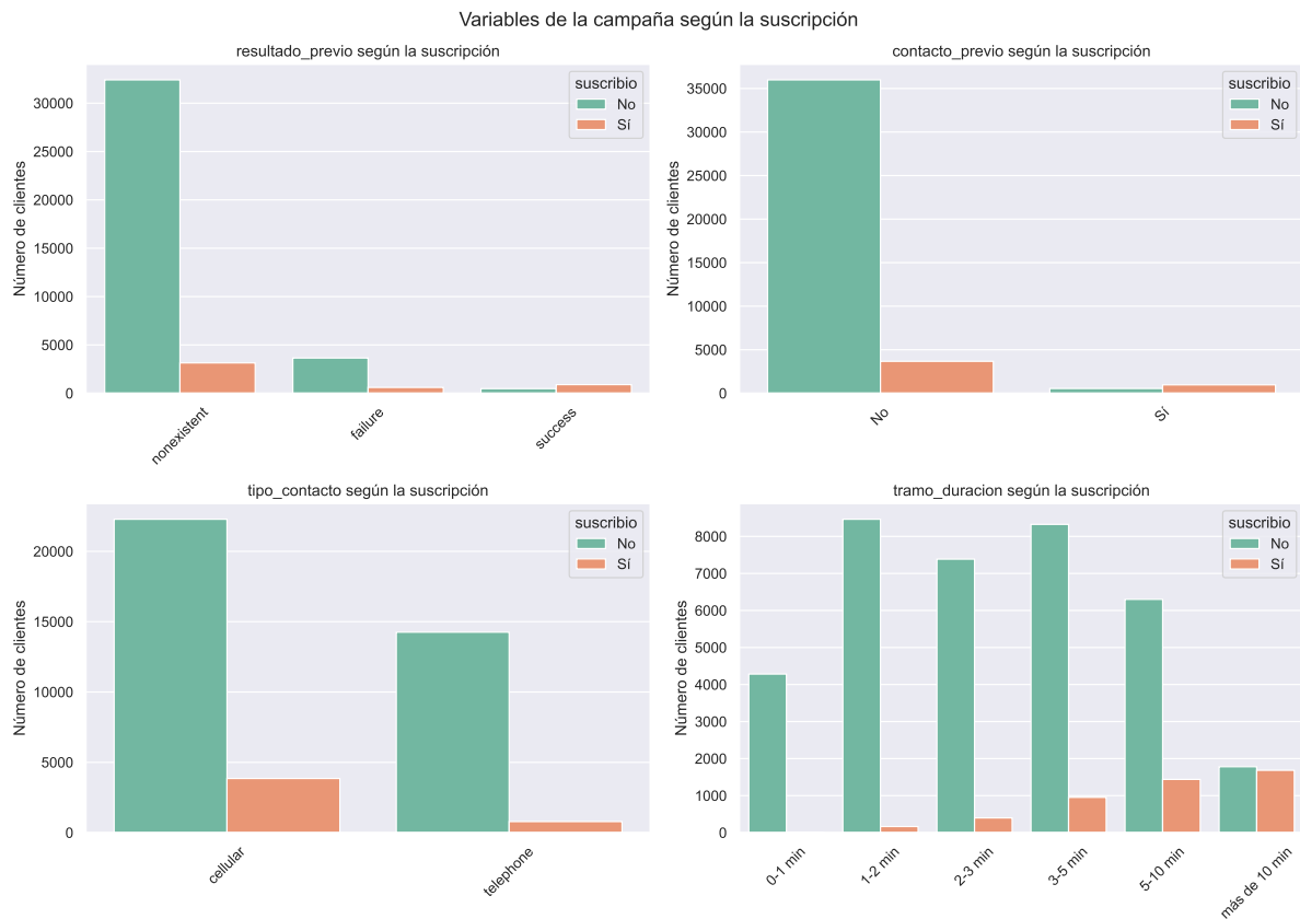
Figura 12: Variables de la campaña según la suscripción.
