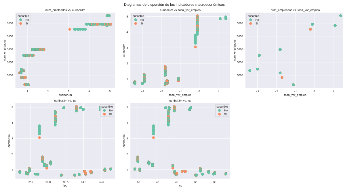
Figura 14: Diagramas de dispersión de los indicadores macroeconómicos.
