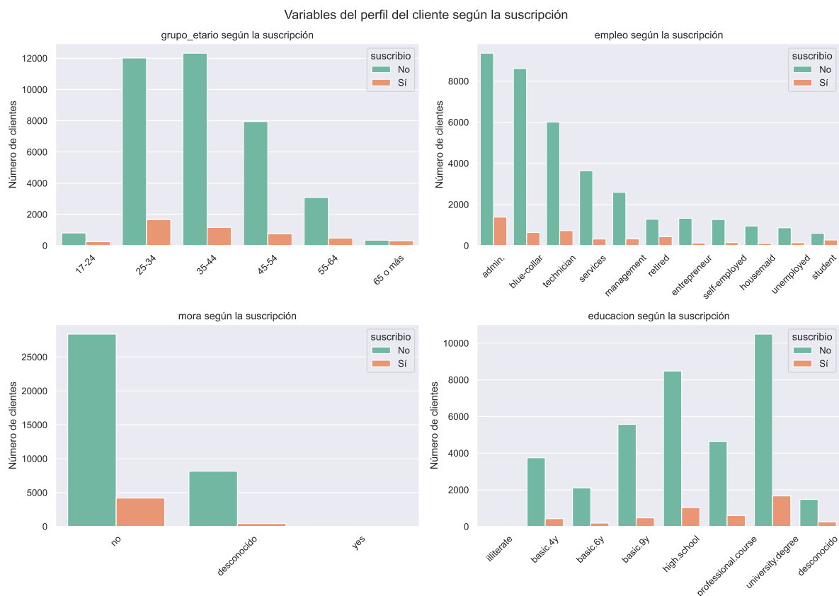
Figura 13: Variables del perfil del cliente según la suscripción.
