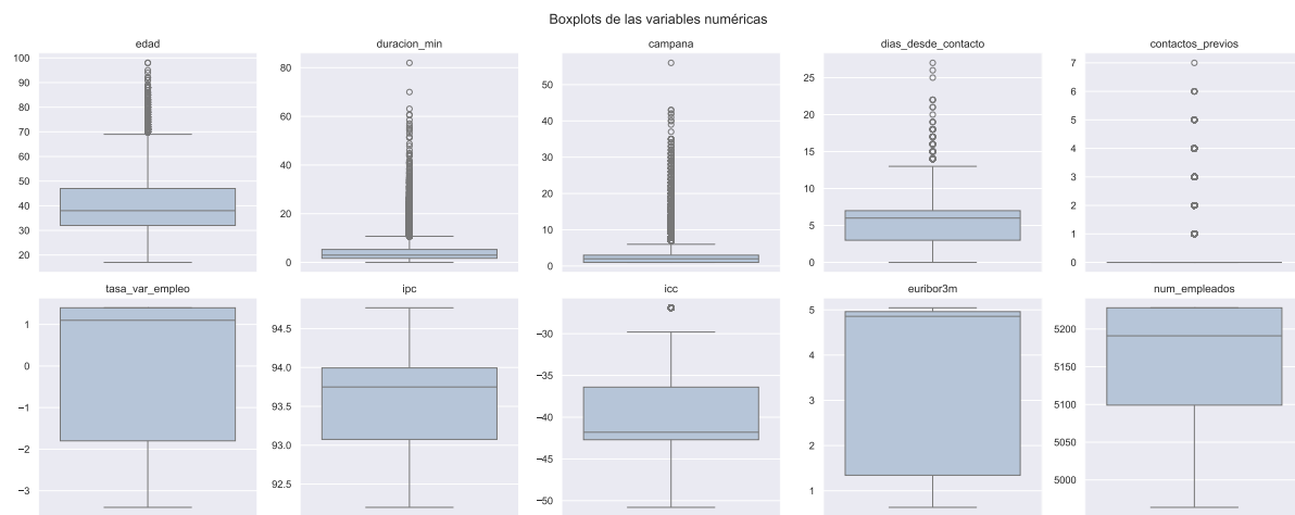
Figura 4: Boxplots de las variables numéricas.
