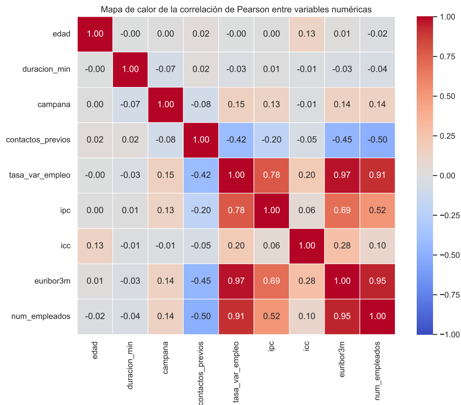
Figura 8: Mapa de calor de la correlación de Pearson entre variables numéricas.
