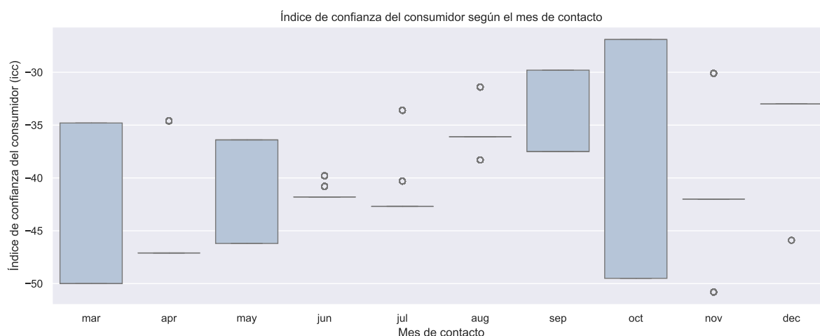
Figura 10: Índice de confianza del consumidor según el mes de contacto.
