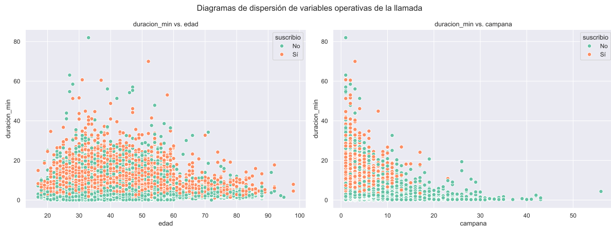
Figura 15: Diagramas de dispersión de variables que describen las llamadas.
