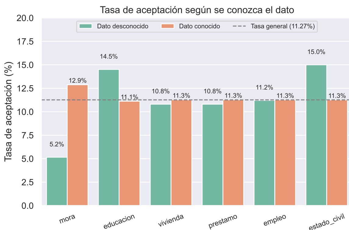
Figura 3: Tasa de aceptación según se conozca el dato.
