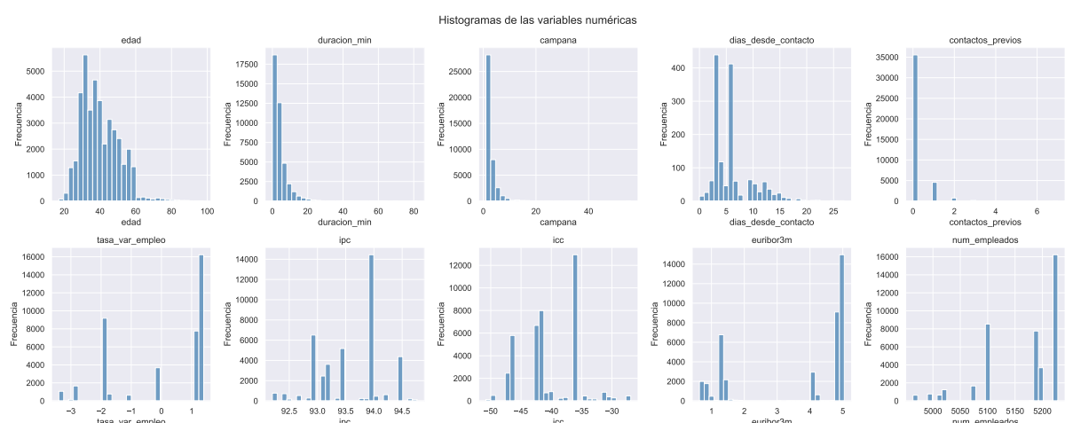
Figura 5: Histogramas de las variables numéricas.
