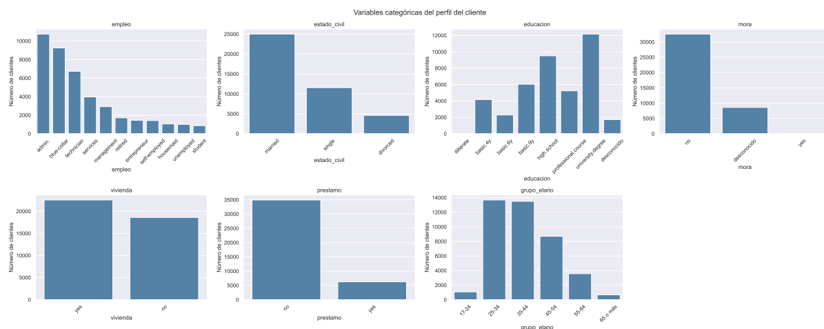
Figura 6: Gráficos de barras de las variables categóricas del perfil del cliente.
