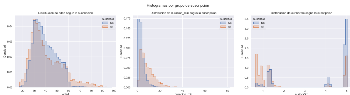
Figura 11: Histogramas de edad, duración y Euribor según la suscripción.
