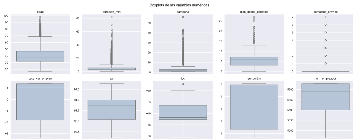
Figura 3: Boxplots de las variables numéricas.
