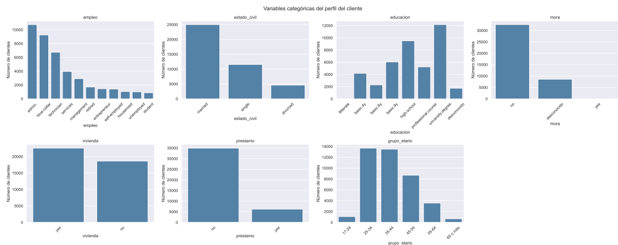
Figura 5: Gráficos de barras de las variables categóricas del perfil del cliente.
