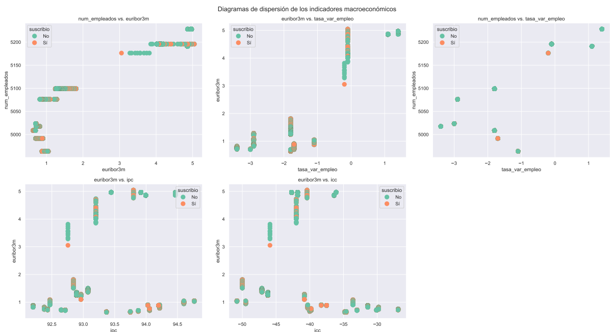
Figura 13: Diagramas de dispersión de los indicadores macroeconómicos.
