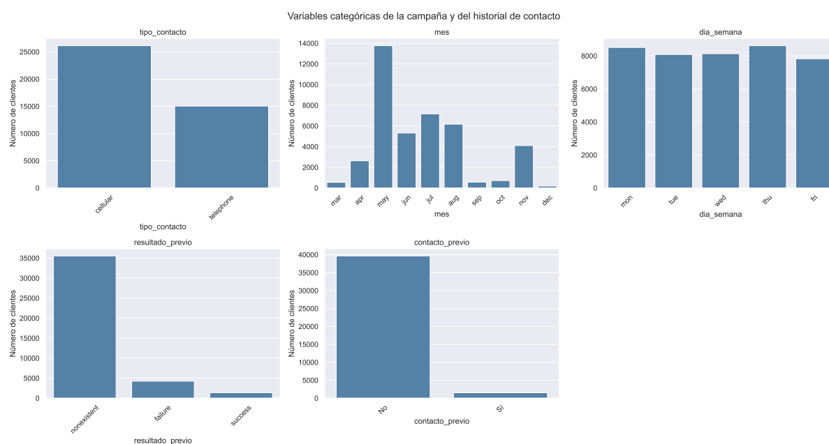
Figura 6: Gráficos de barras de las variables categóricas de la campaña y del historial de contacto.
