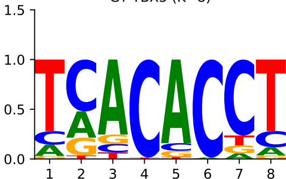
GT TBX5 (K=8)
