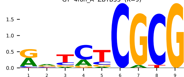
GT 4f6n_A ZBTB33 (K=9)
