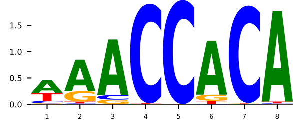
GT 410z_A RUNX1 (K=8)
