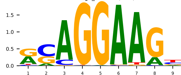
GT 6vge_A ERG (K=9)
