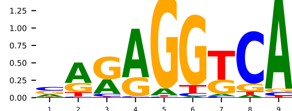
GT 6fbr_B RXRA (K=9)
