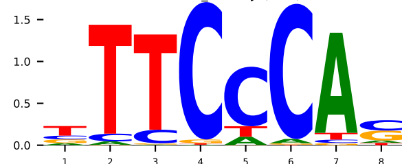
GT 6dks_G RBPJ (K=8)
