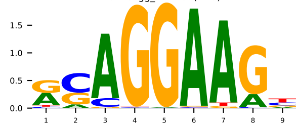
GT 6vvg_A ERG (K=9)
