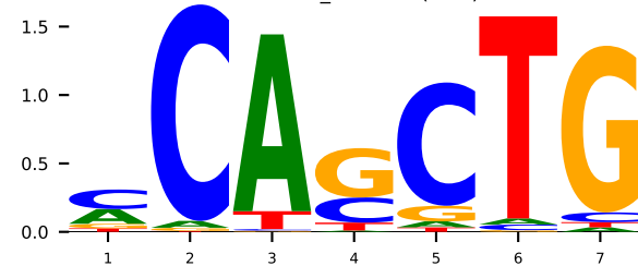
GT 6od3_B TCF4 (K=7)
