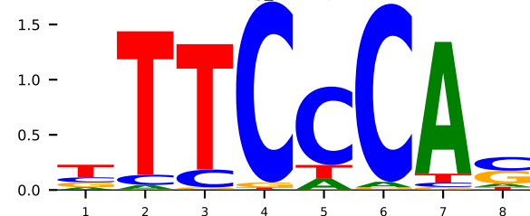
GT 3iag_C RBPJ (K=8)
