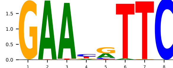
GT 7dcj_B HSF1 (K=8)
