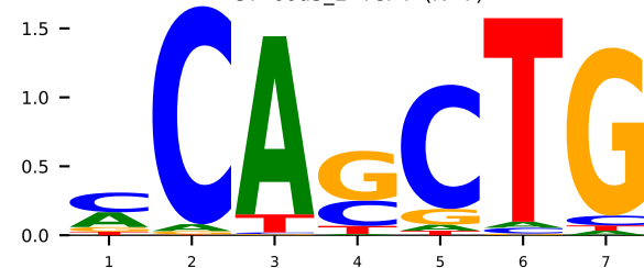
GT 6od3_E TCF4 (K=7)
