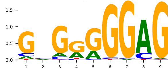
GT 5kl4_A WT1 (K=9)
