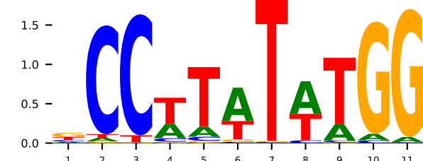
GT 1srs_A SRF (K=11)
