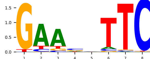
GT 7dcj_A HSF1 (K=8)
