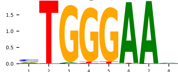
GT 3v79_C RBPJ (K=8)
