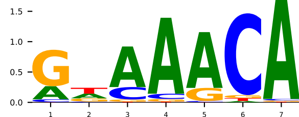
GT 6lbi_K FOXO1 (K=7)
