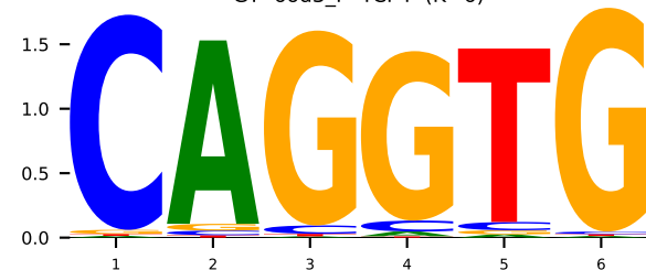
GT 6od3_F TCF4 (K=6)
