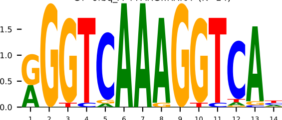
GT 6fbq_A PPARG::RXRA (K=14)
