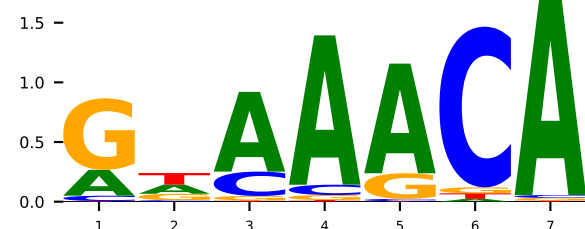
GT 6lbi_L FOXO1 (K=7)
