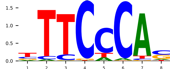
GT 6dks_C RBPJ (K=8)
