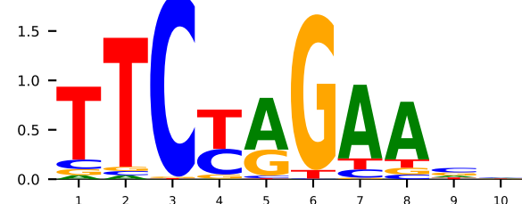
GT 5hdn_A HSF1 (K=10)
