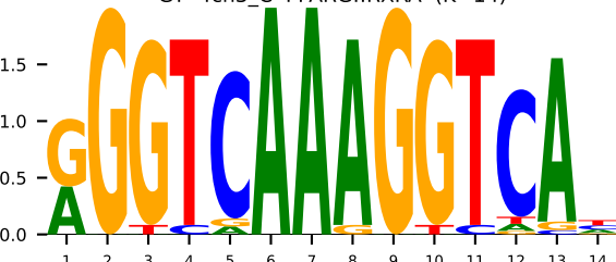
GT 4cn3_C PPARG::RXRA (K=14)
