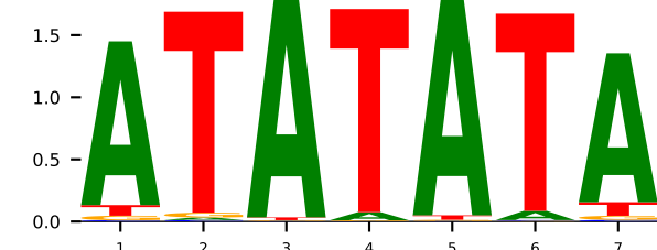
GT 7oh9_K SPT15 (K=7)
