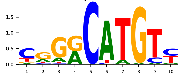
GT 2ady_A TP53 (K=10)
