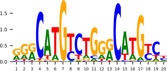
GT 6fj5_D P53 (K=20)
