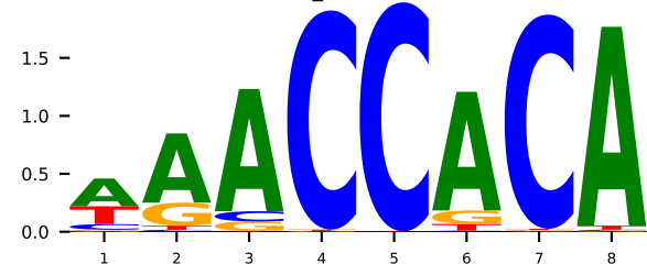
GT 3wts_F RUNX1 (K=8)
