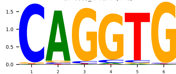
GT 6od3_A TCF4 (K=6)
