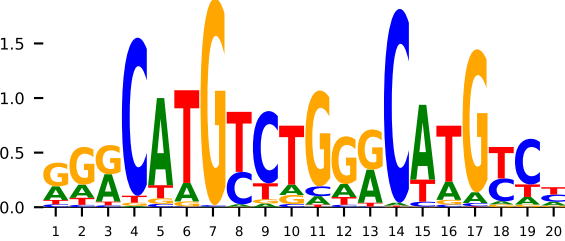
GT 6fj5_C P53 (K=20)
