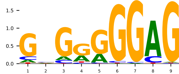
GT 6b0q_A WT1 (K=9)
