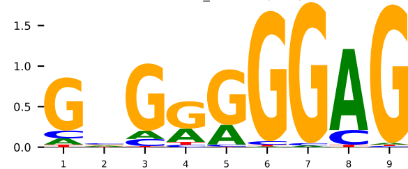
GT 5kl4_D WT1 (K=9)
