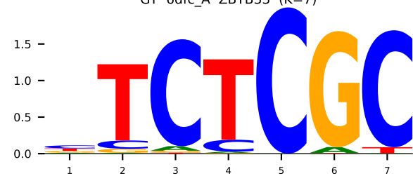
GT 6dfc_A ZBTB33 (K=7)
