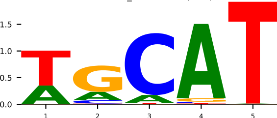
GT 1e3o_C POU2F1 (K=5)
