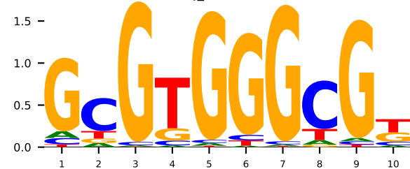
GT 4x9j_A EGR1 (K=10)
