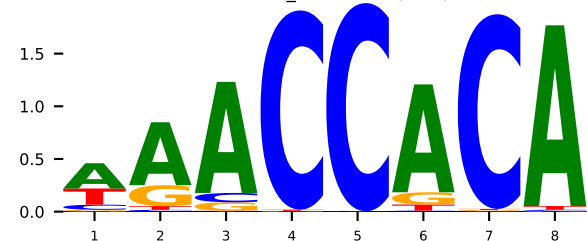
GT 3wtw_F RUNX1 (K=8)
