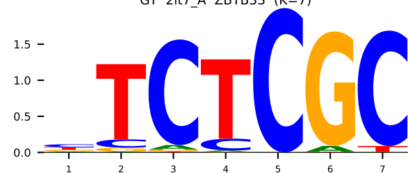
GT 2lt7_A ZBTB33 (K=7)
