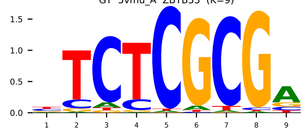
GT 5vmu_A ZBTB33 (K=9)
