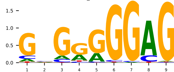
GT 5kl3_A WT1 (K=9)
