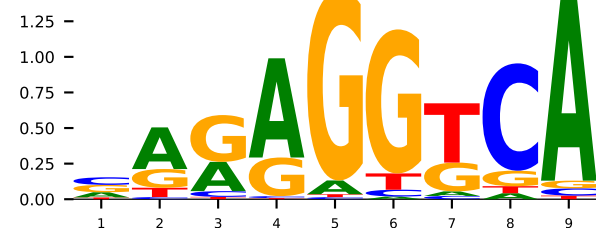
GT 4cn3_D RXRA (K=9)
