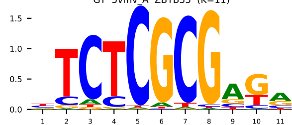
GT 5vmv_A ZBTB33 (K=11)
