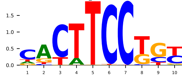
GT 3wts_C ETS1 (K=10)
