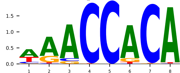
GT 3wtu_A RUNX1 (K=8)
