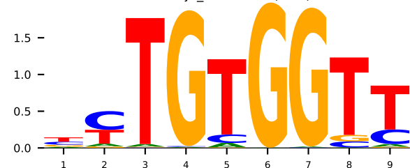
GT 1hjb_F RUNX1 (K=9)
