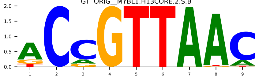
GT ORIG_ZNF385D.M09365_1.94d
