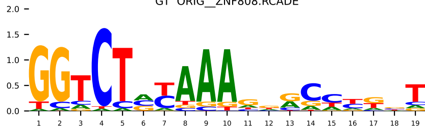
GT 6e8c_A_DUX4.MA0468.1
