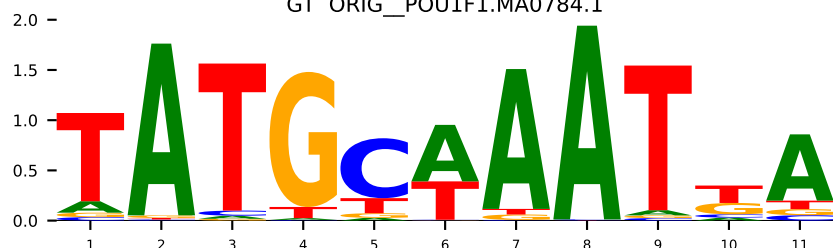
GT ORIG_AR.M05563_1.94d
