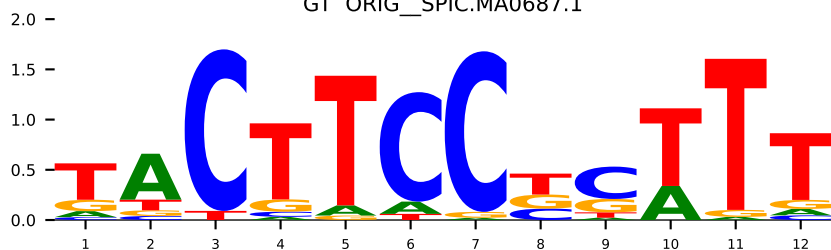
GT ORIG_SPIC.MA0687.1
