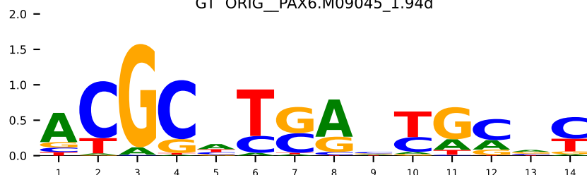
GT 1mdm_A_PAX5.PAX5_HUMAN.H11MO.0.A
