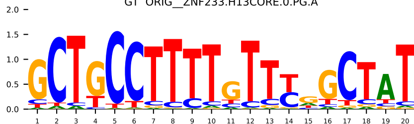
GT ORIG_ZNF233.H13CORE.0.PG.A
