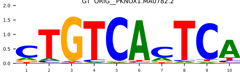
GT ORIG_PKNOX1.MA0782.2
