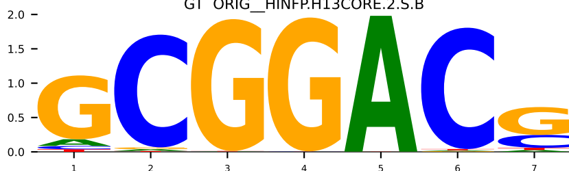
GT ORIG_HINFP.H13CORE.2.S.B
