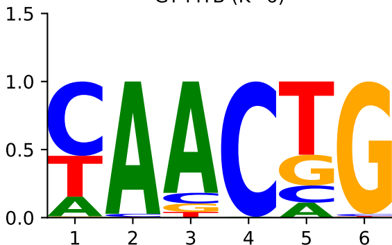
GT MYB (K=6)
