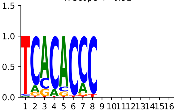
TFScope r=0.51
