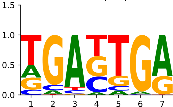
GT PBX1 (K=7)
