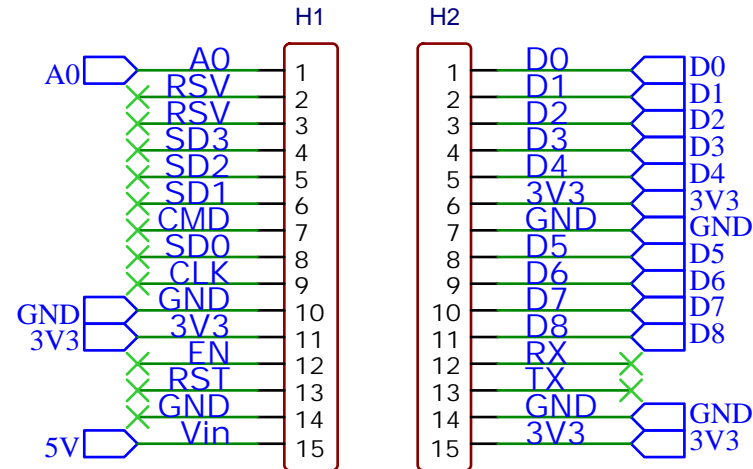
NodeMCU
