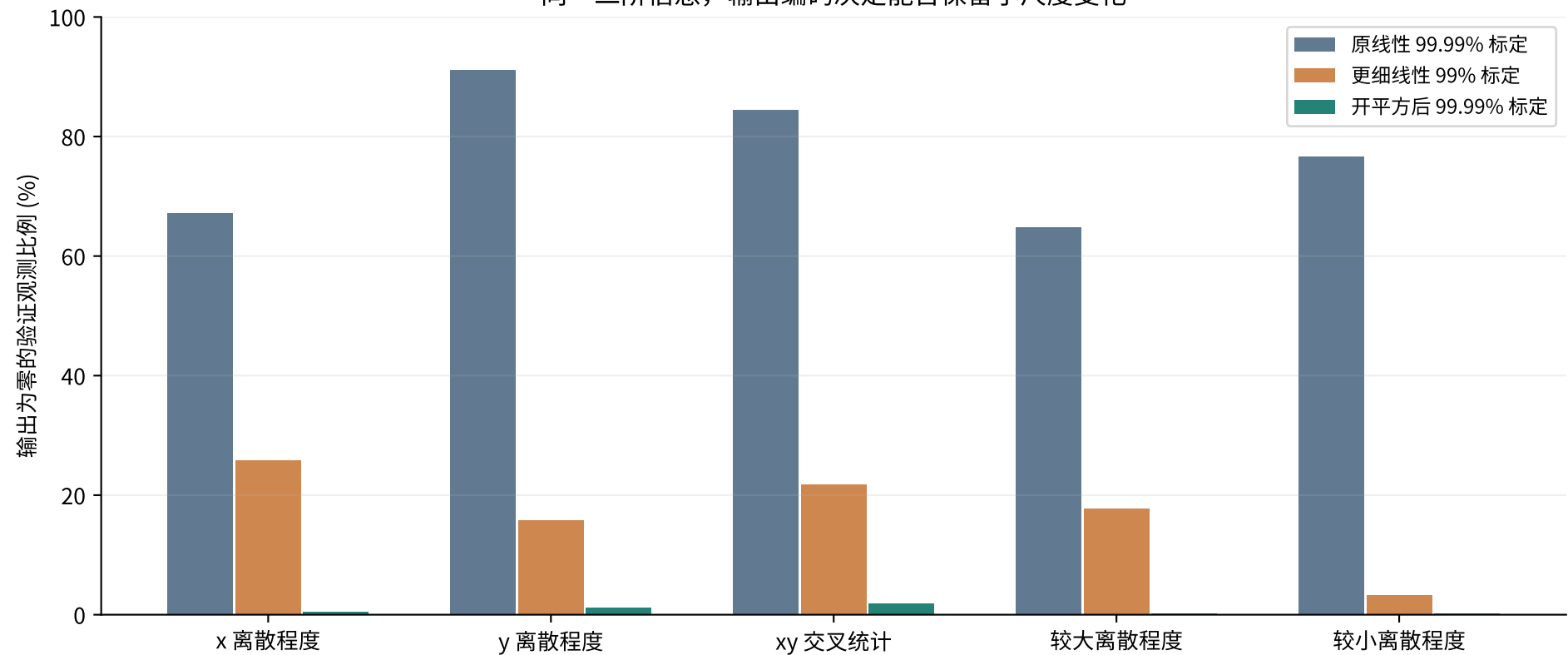
同一二阶信息，输出编码决定能否保留小尺度变化
