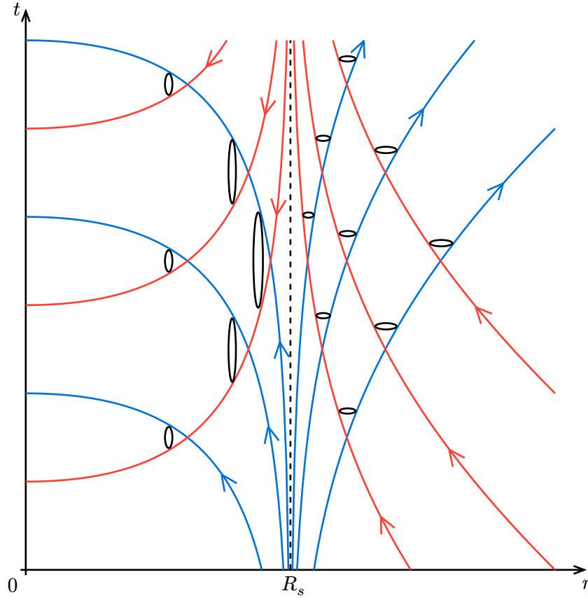
Fig. 2. – Structure des cônes de lumière (seul le coté future est montré) pour la métrique de Schwarzschild en bleu les rayons sortants, et en rouge les rayons entrants
