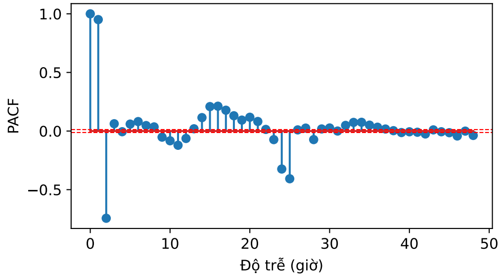
PACF của phụ tải (lag 0-48)
