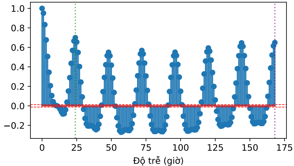
ACF của phụ tải (lag 0-168)
