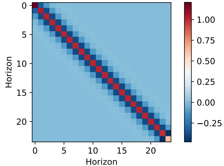
Mã trận chính xác W (đã shrink, \text{cond} \leq 150 )
