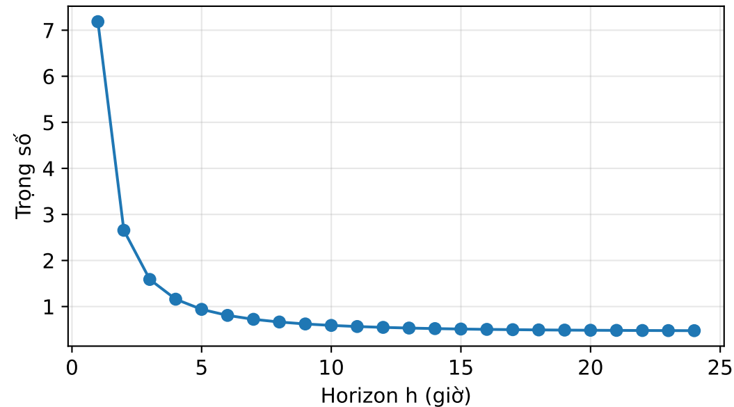
Trọng số nghịch phương sai w_h^{invvar} theo horizon
