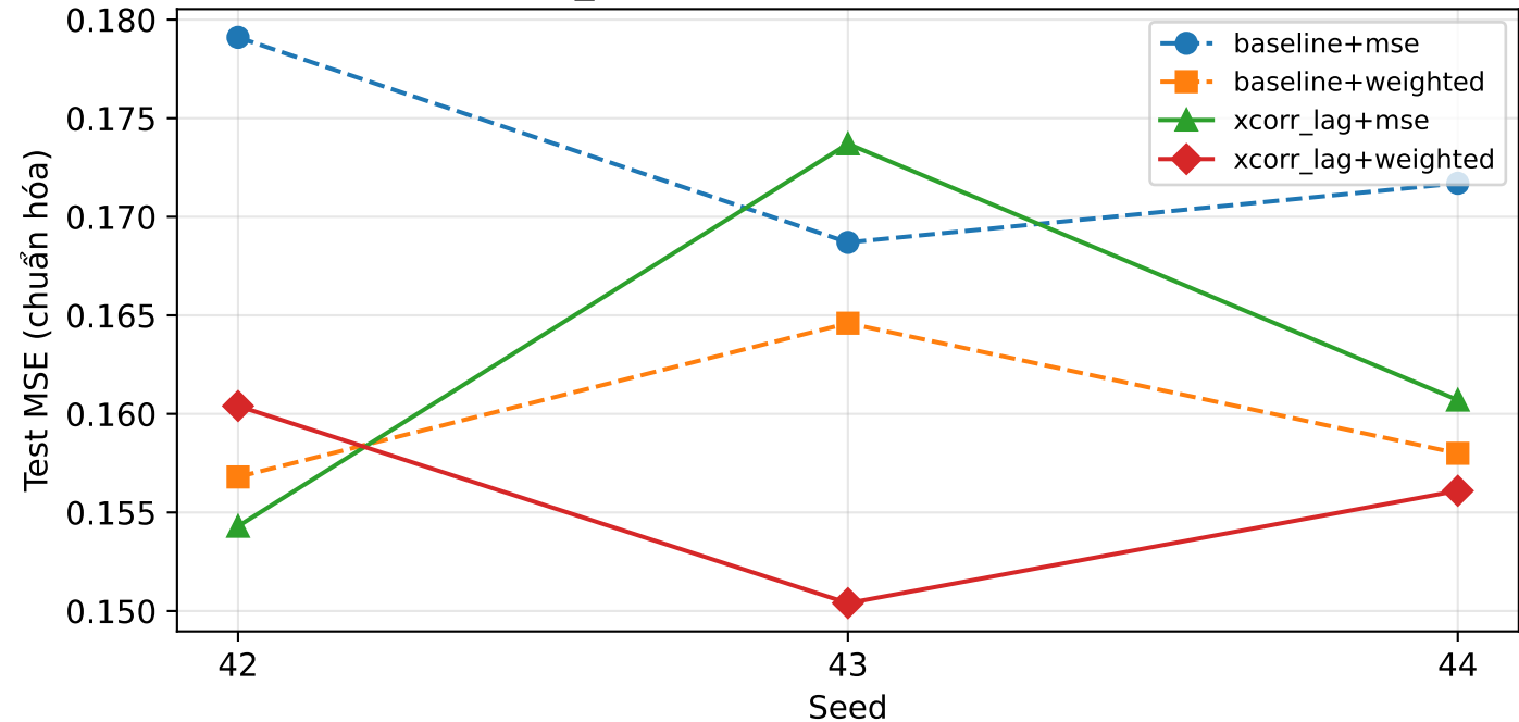
MSE theo từng seed: xcorr\_lag+mse biến động mạnh (seed 43 kém hơn baseline)
