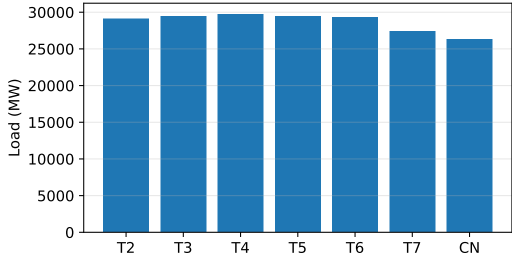
Phụ tải trung bình theo ngày trong tuần
