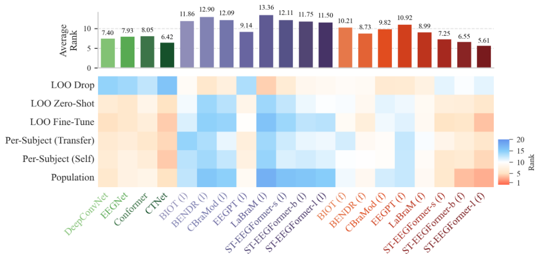
Rangs moyens du benchmark ST-EEGFormer
