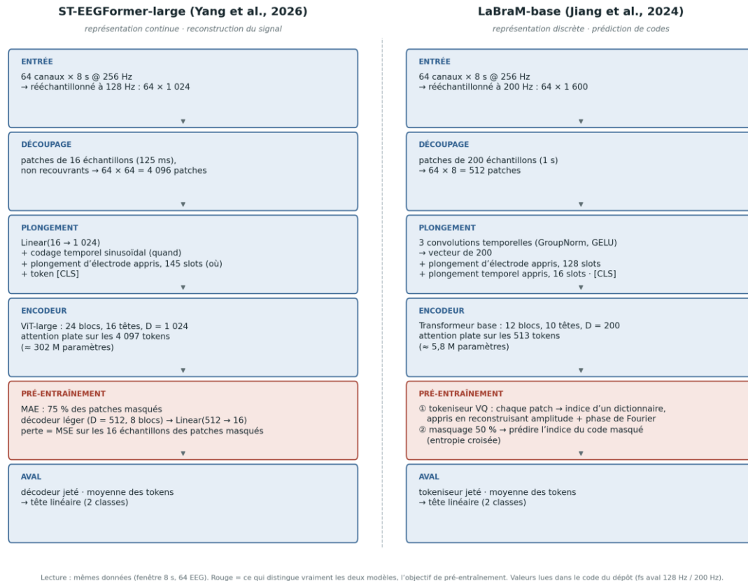
Figure 3.2. ST-EEGFormer-large et LaBraM-base, étape par étape, sur une même fenêtre de 8 s à 64 canaux. En rouge, la seule étape où les deux modèles diffèrent fondamentalement : l'objectif de pré-entraînement. Valeurs lues dans le code du dépôt.
