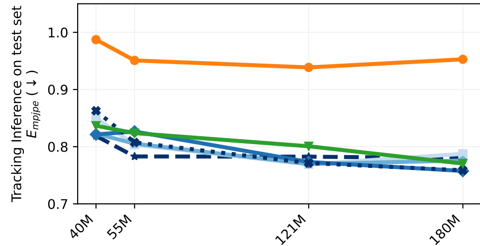
Model: MLP
