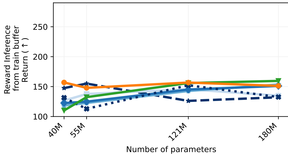
Model: MLP
