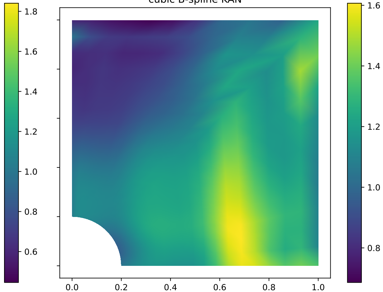
cubic B-spline KAN
