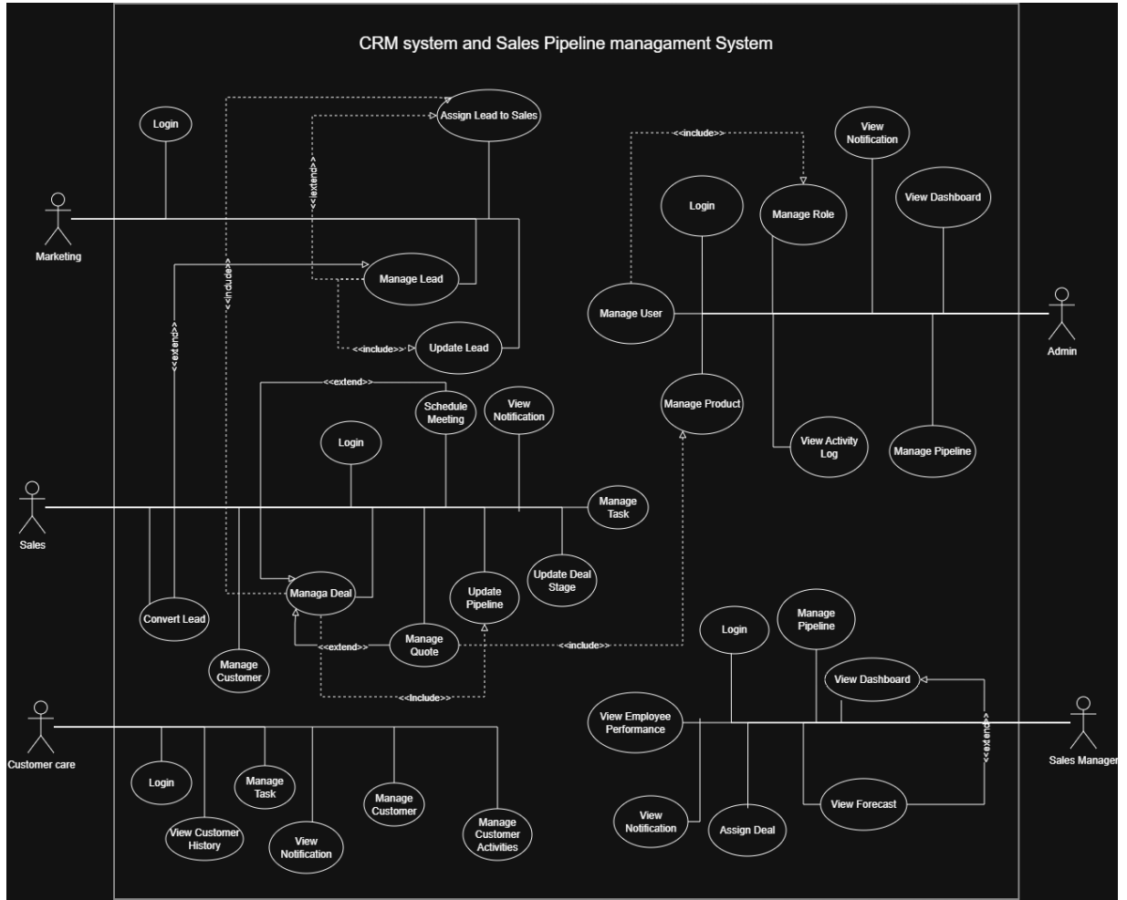
Hình 3.1: Use Case Diagram
