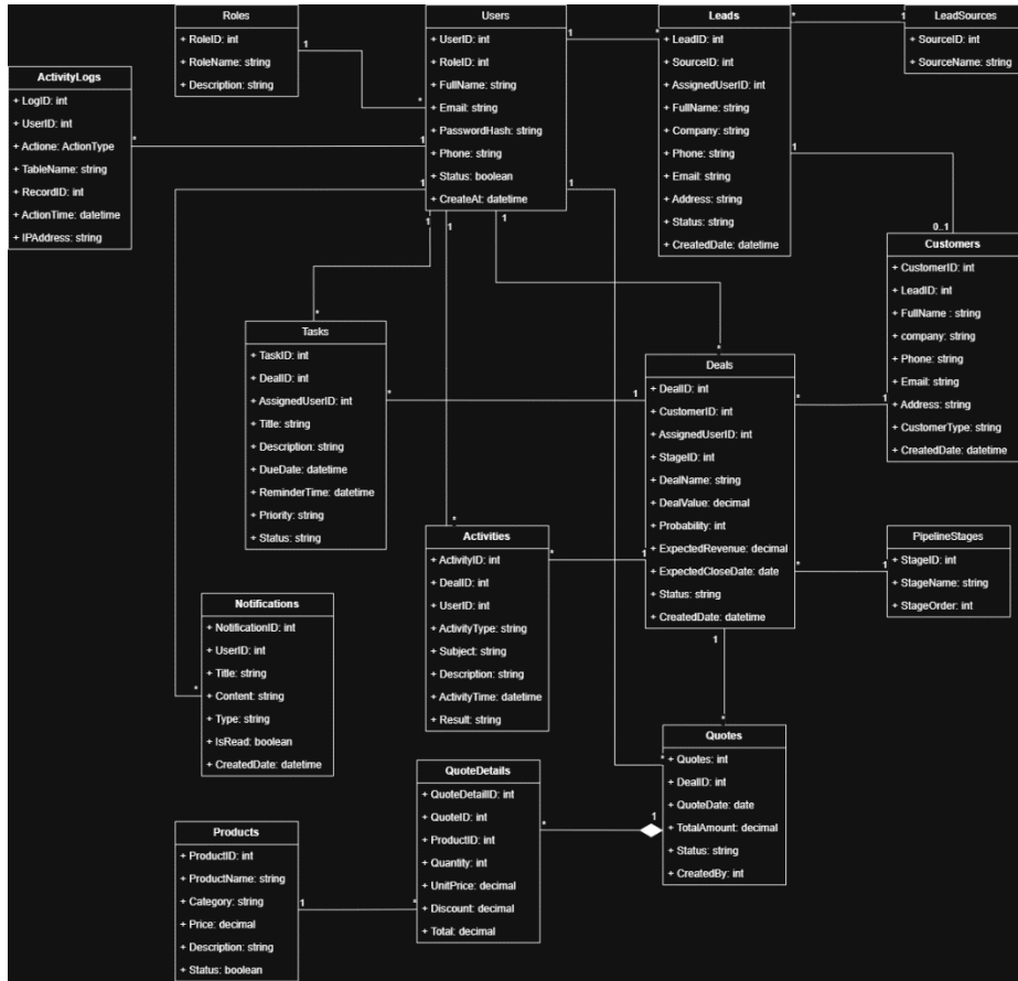
Hình 3.10: Class Diagram
