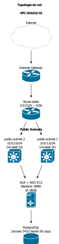
Figure 17: Topología de red en AWS
