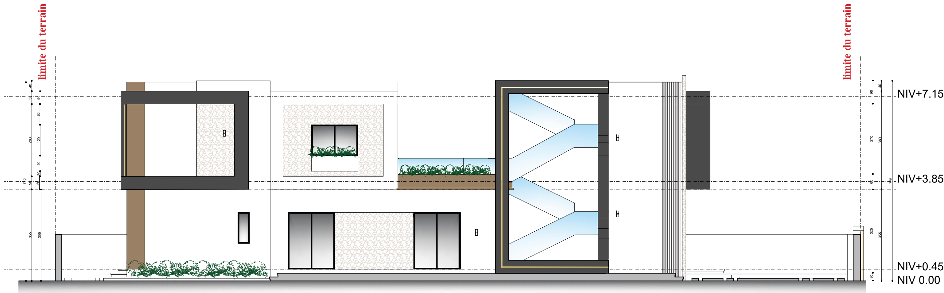
FAÇADE OUEST
