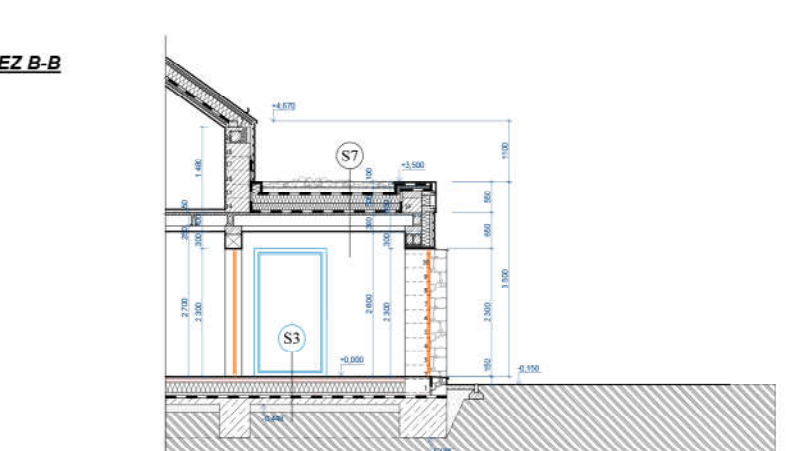
REZ B-B
