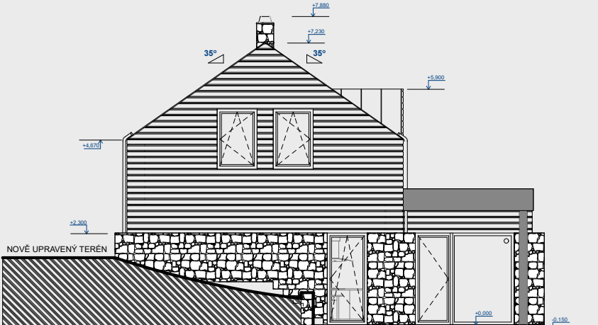
POHLED ZÁPADNÍ
