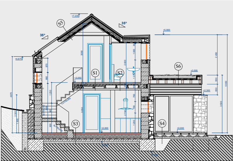
ŘEZ A-A
