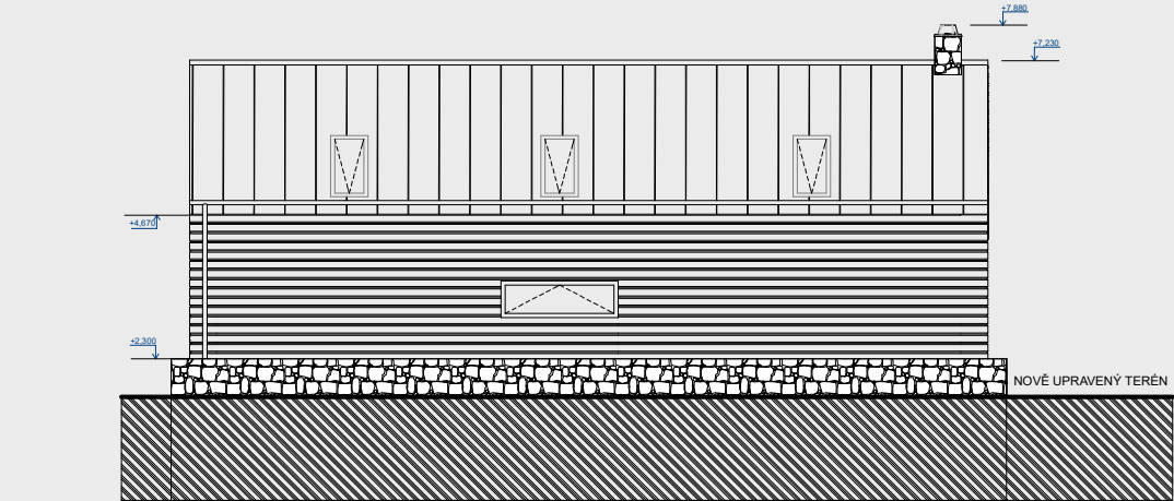
POHLED SEVERNÍ
