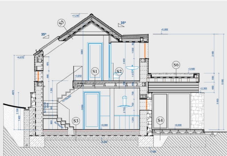
ŘEZ A-A
