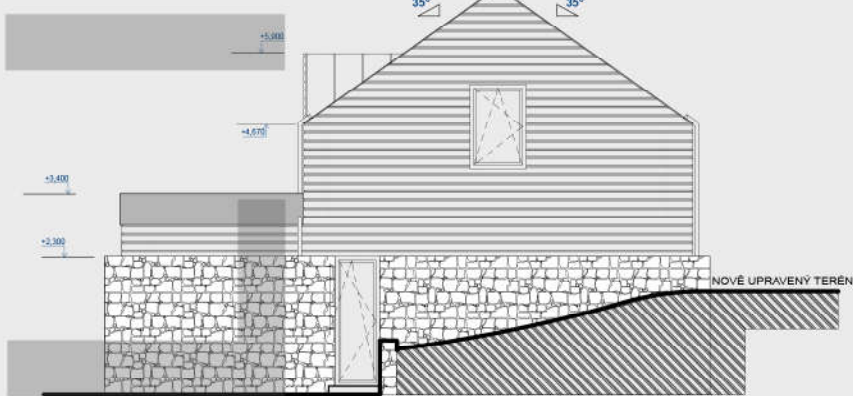
POHLED VÝCHODNÍ
