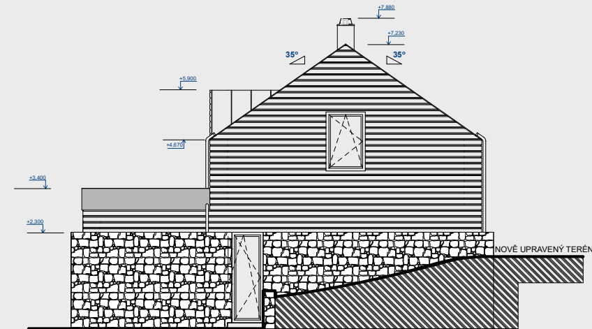
POHLED VÝCHODNÍ
