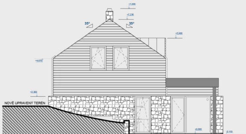
POHLED ZÁPADNÍ
