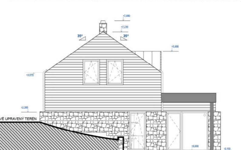
POHLED ZÁPADNÍ
