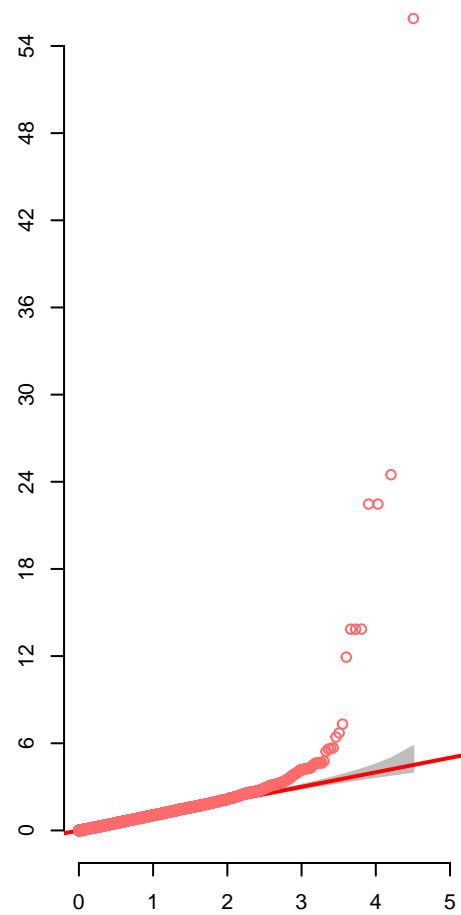
FarmCPU.FHBZEA
