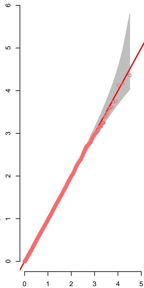
FarmCPU.FHBDISIND
