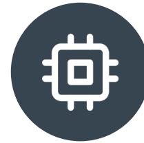
IA generativa
