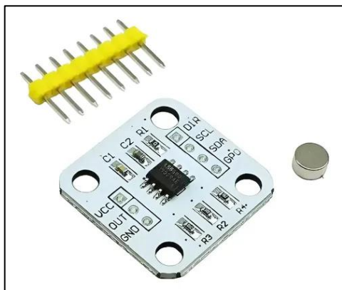
Imagen 47 – Encoder AS5600
