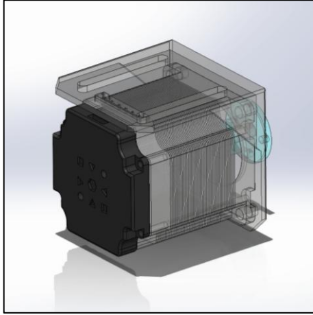
Imagen 35 – Porta Encoder.
