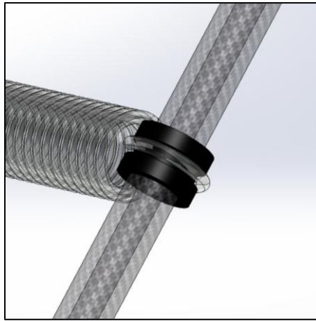
Imagen 37 – Porta resortes.
