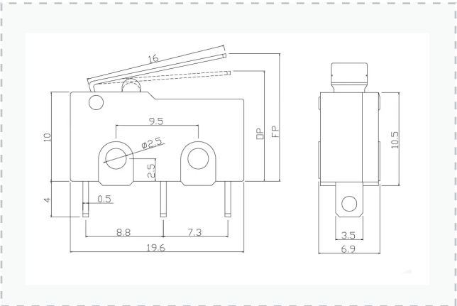
Plano Dimensional / Cotas (mm)
