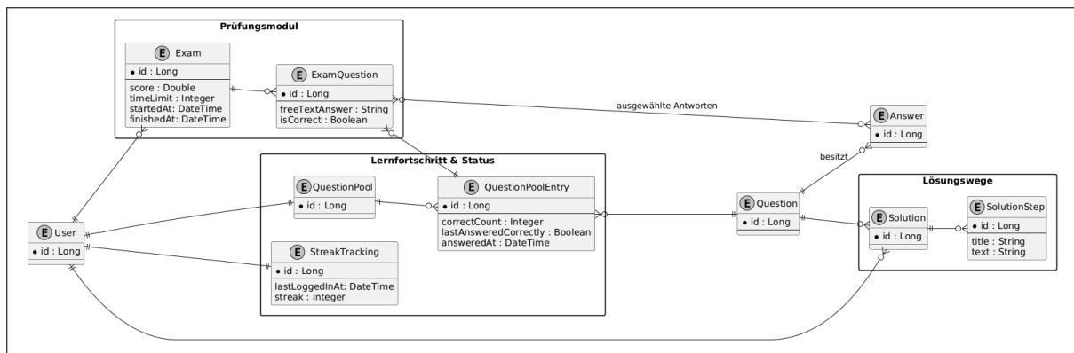
Abbildung 40: Für dieses Teilprojekt relevanter Ausschnitt des Datenbankmodells der Anwendung
