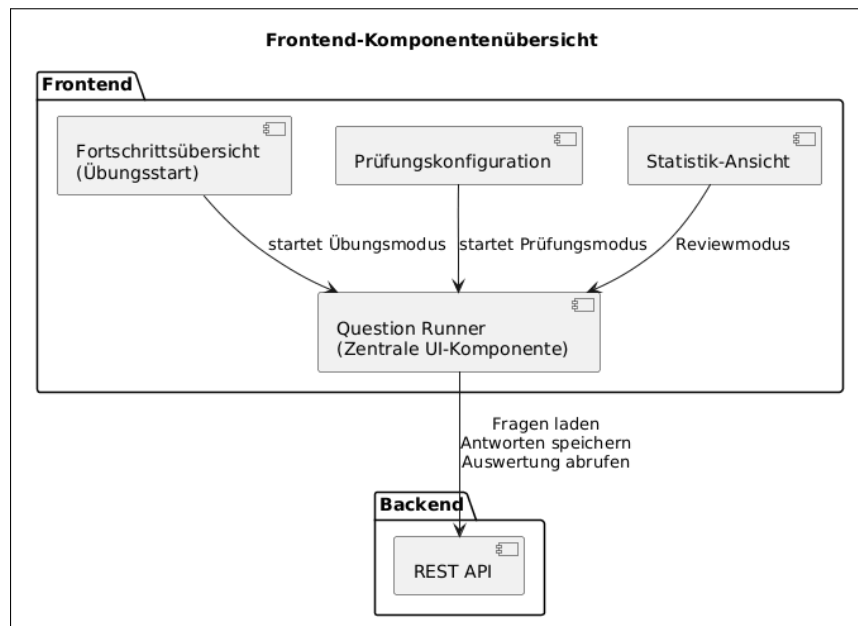
Abbildung 38: Komponentendiagramm des Frontends
