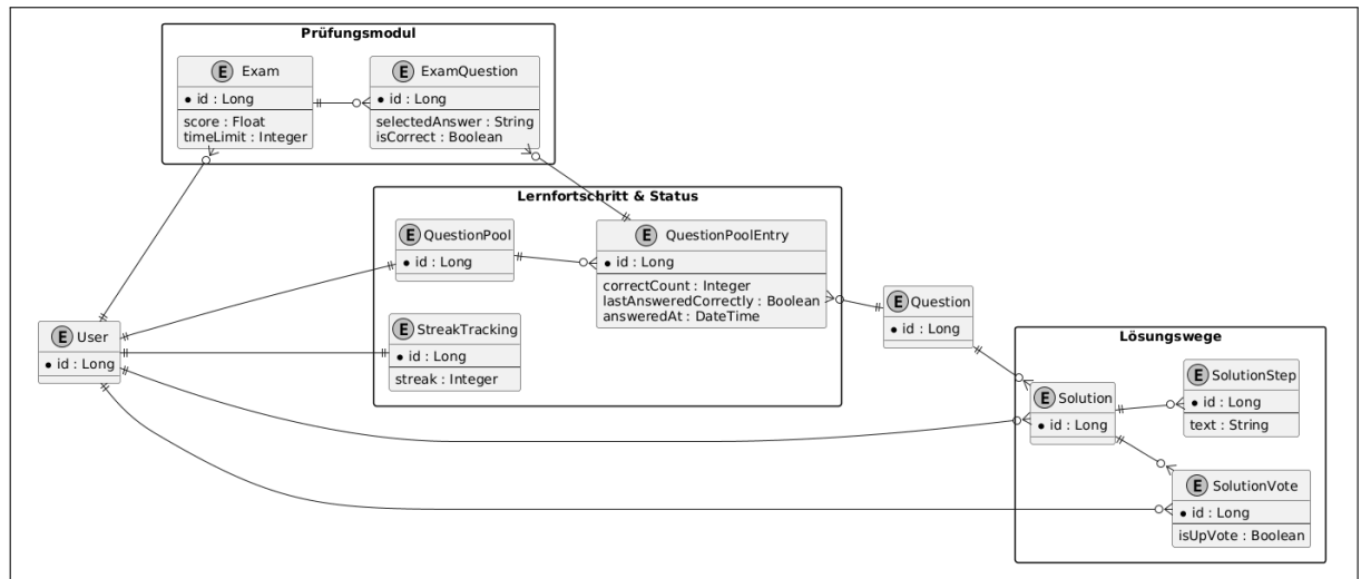
Abbildung 36: Datenbankmodell der Anwendung
