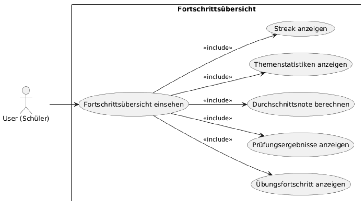
Abbildung 7: Use-Case Diagramm: Fortschrittsübersicht
