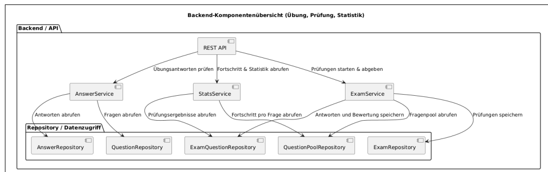
Abbildung 24: Komponentendiagramm des Backends
