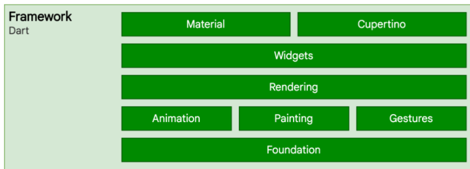
Abbildung 10: Schichtenmodell der Flutter-Architektur [49]
