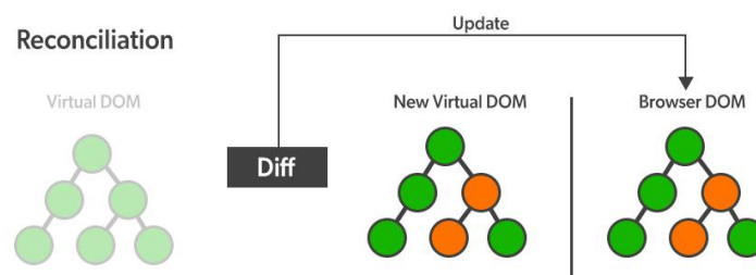
Abbildung 12: Vergleich zwischen Real DOM und Virtual DOM beim Diffing-Prozess [?]
