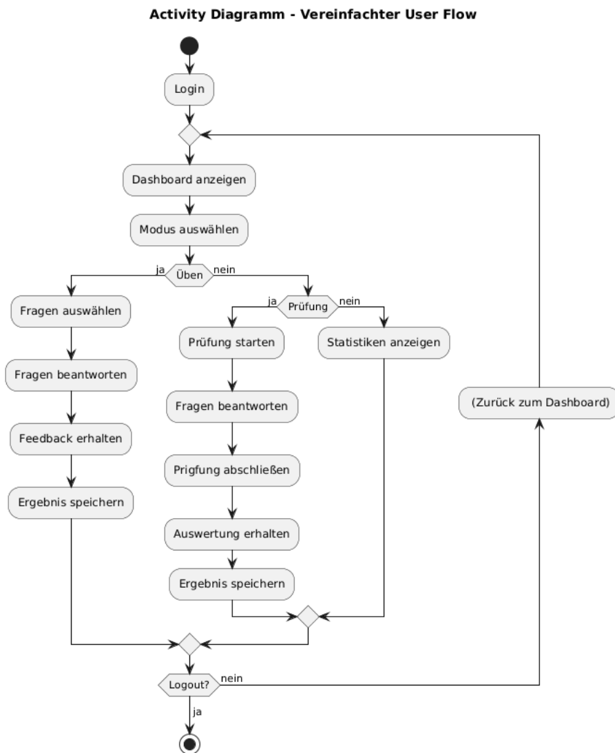
Abbildung 13: Ablaufdiagramm eines Users [59]
