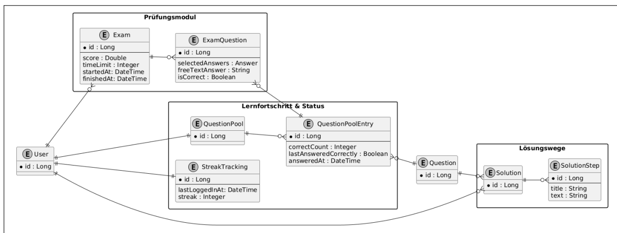
Abbildung 40: Für dieses Teilprojekt relevanter Ausschnitt des Datenbankmodells der Anwendung
