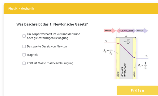
(a) Multiple-Choice-Frage
