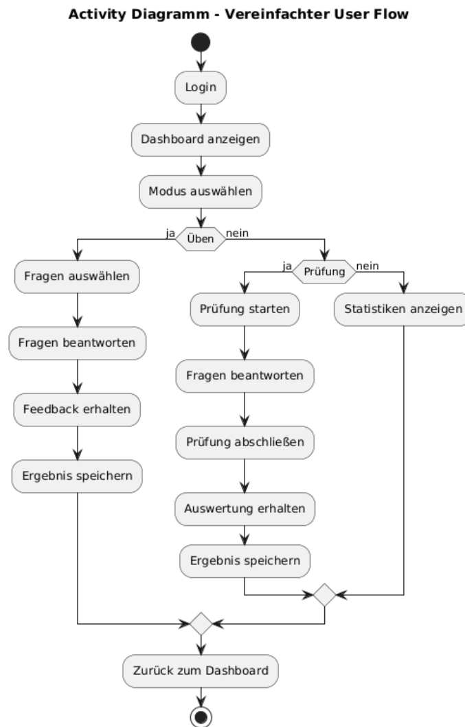
Abbildung 7: Ablaufdiagramm eines Users [11]
