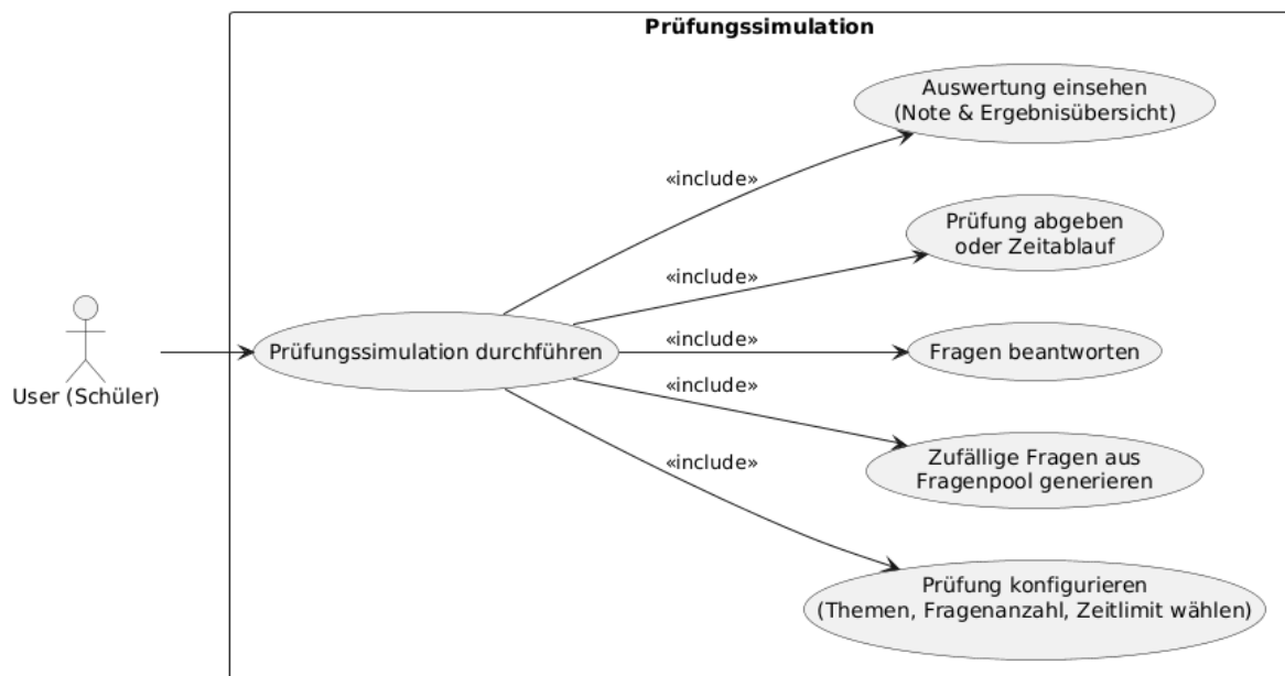
Abbildung 9: Use-Case Diagramm: Prüfungsmodus [11]
