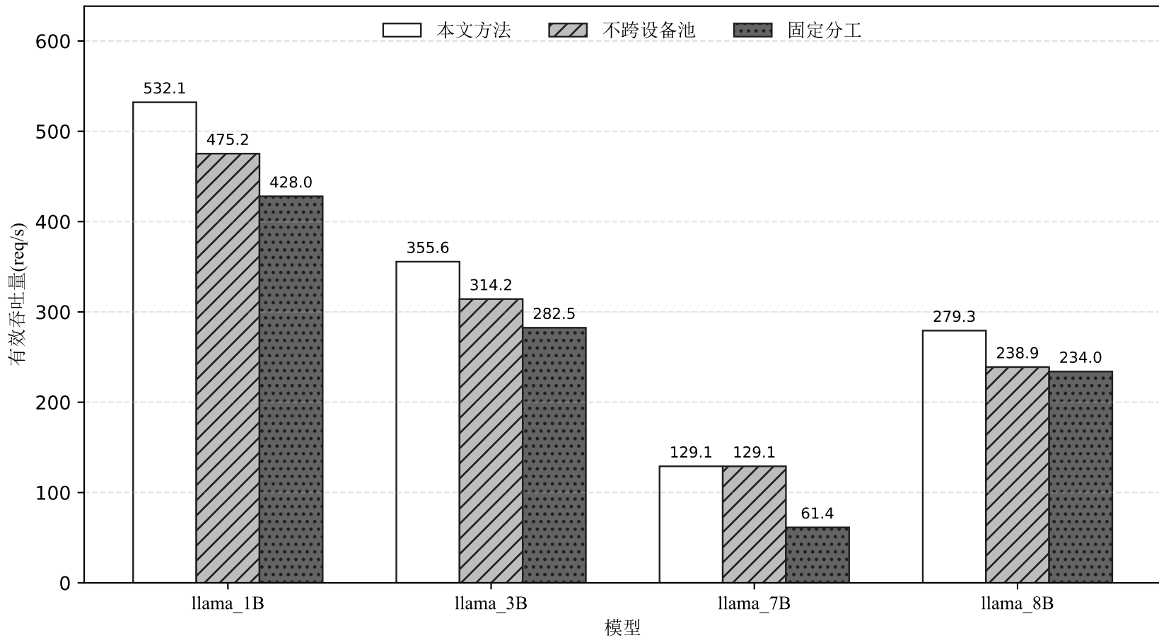
有效吞吐量对比图
